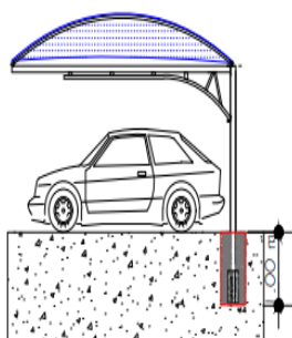
03 Vista Lateral
