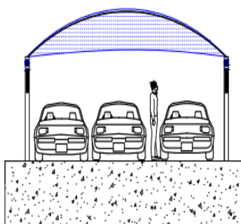
02 Vista Frontal
