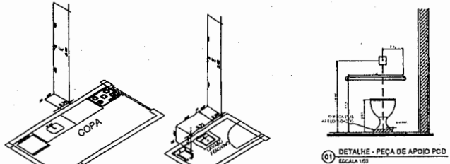
02 PROJETO HIDRÁULICO
