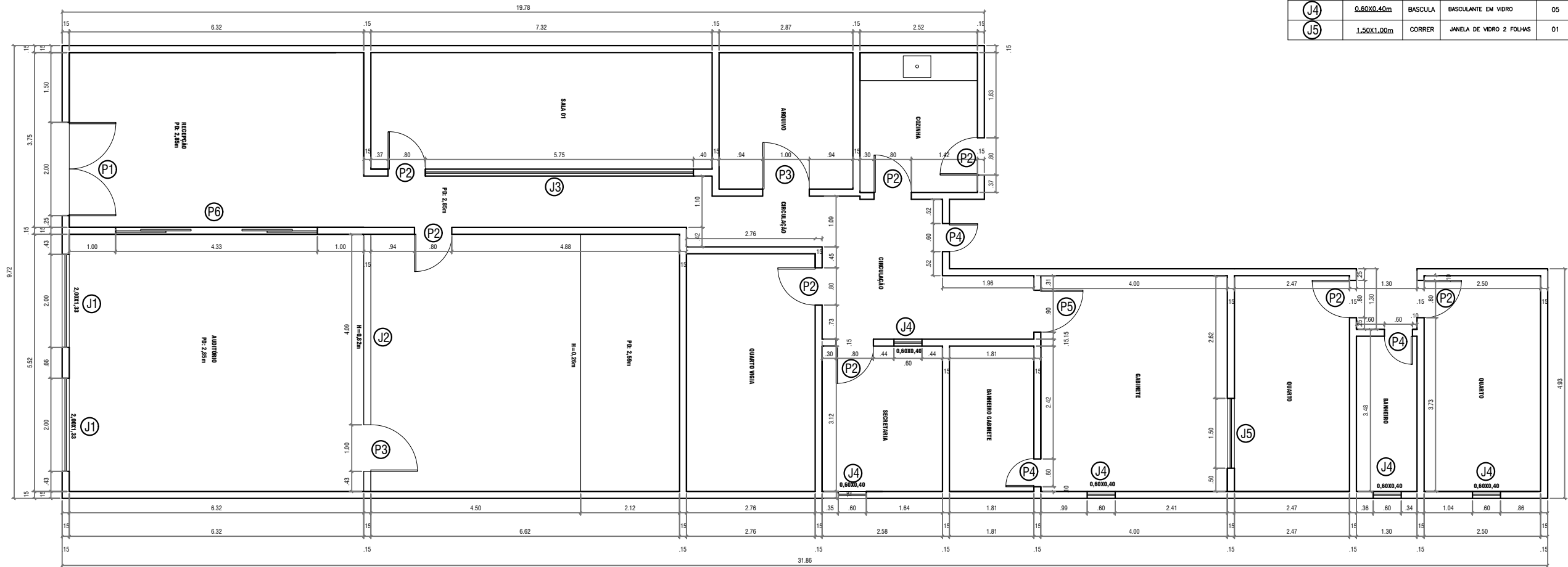
PLANTA BAIXA ESCALA 1:100
