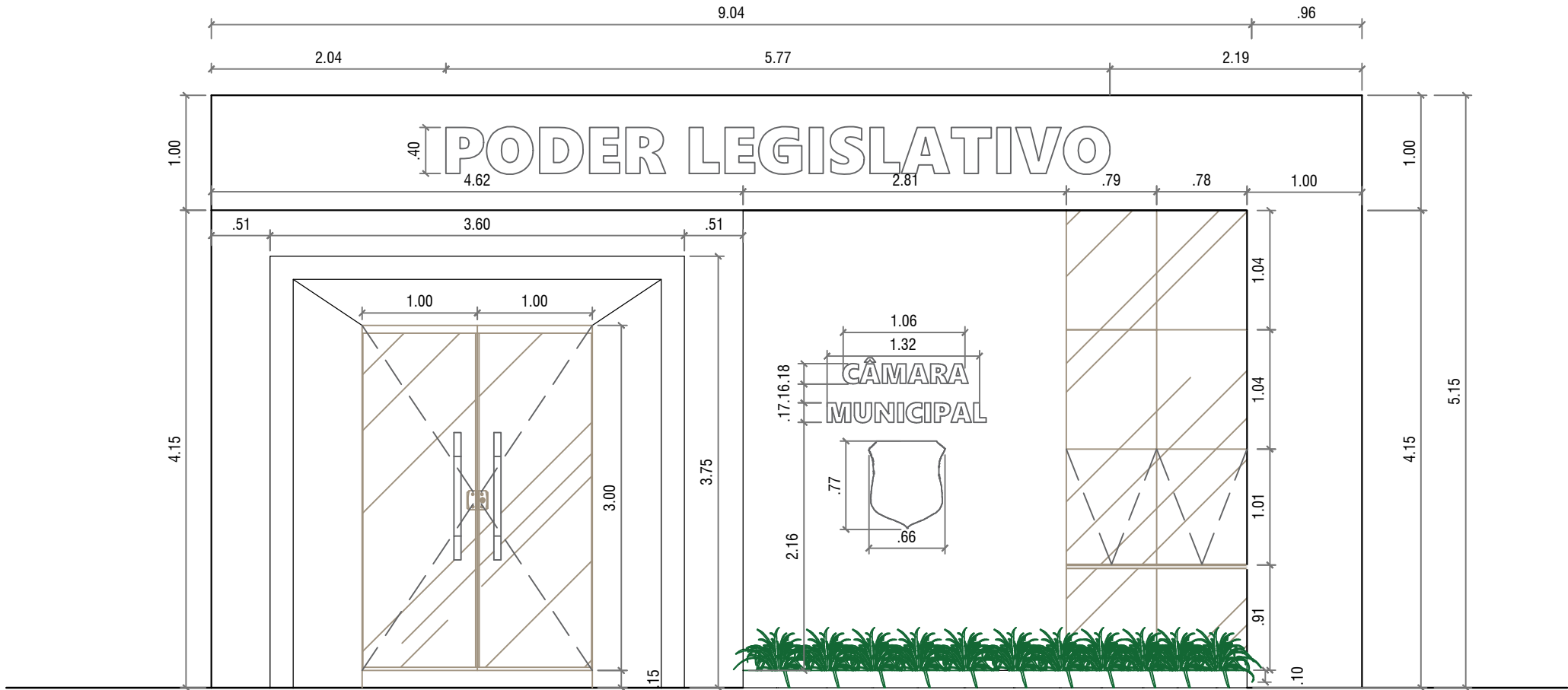
VISTA DE FACHADA - MEDIDAS ESCALA 1:50
