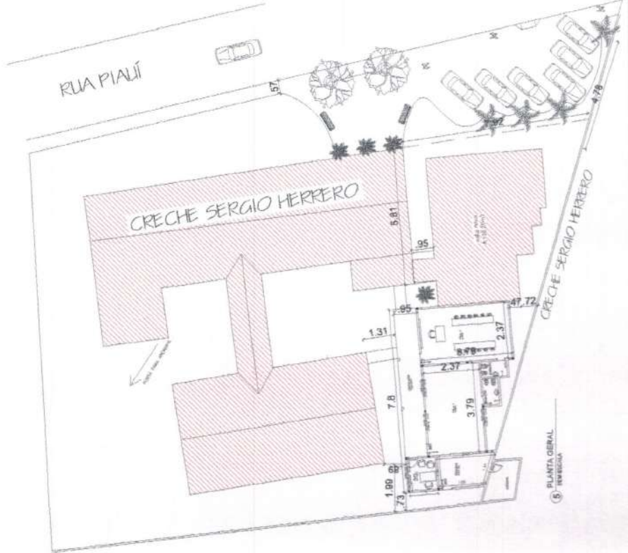
2 PLANTA COBERTURA 1:100
