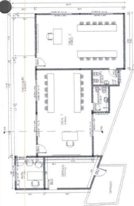
1 PLANTA BAIXA 1:100 A/144.40m2
