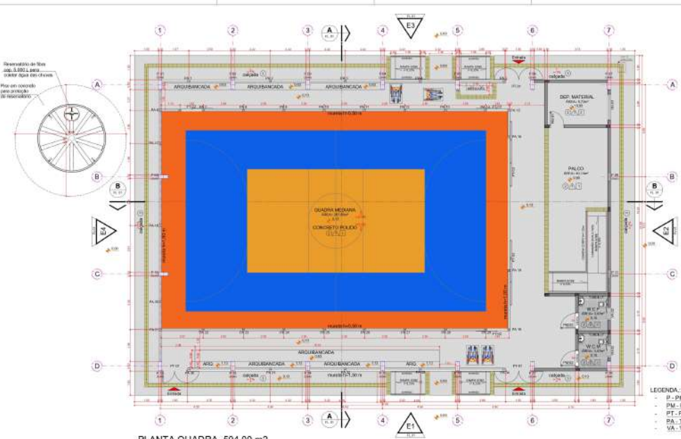
PLANTA QUADRA 504,00 m 2 Escala 1:75 OBS: As demarcações a serem executadas no piso não correspondem as medidas oficiais.
