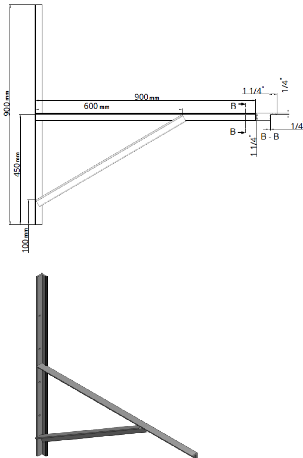
Figura 4 - Desenho técnico da cantoneira/suportes C4, destinada a unidades condensadoras com capacidade na faixa de 48.000 a 60.000 BTU/h
