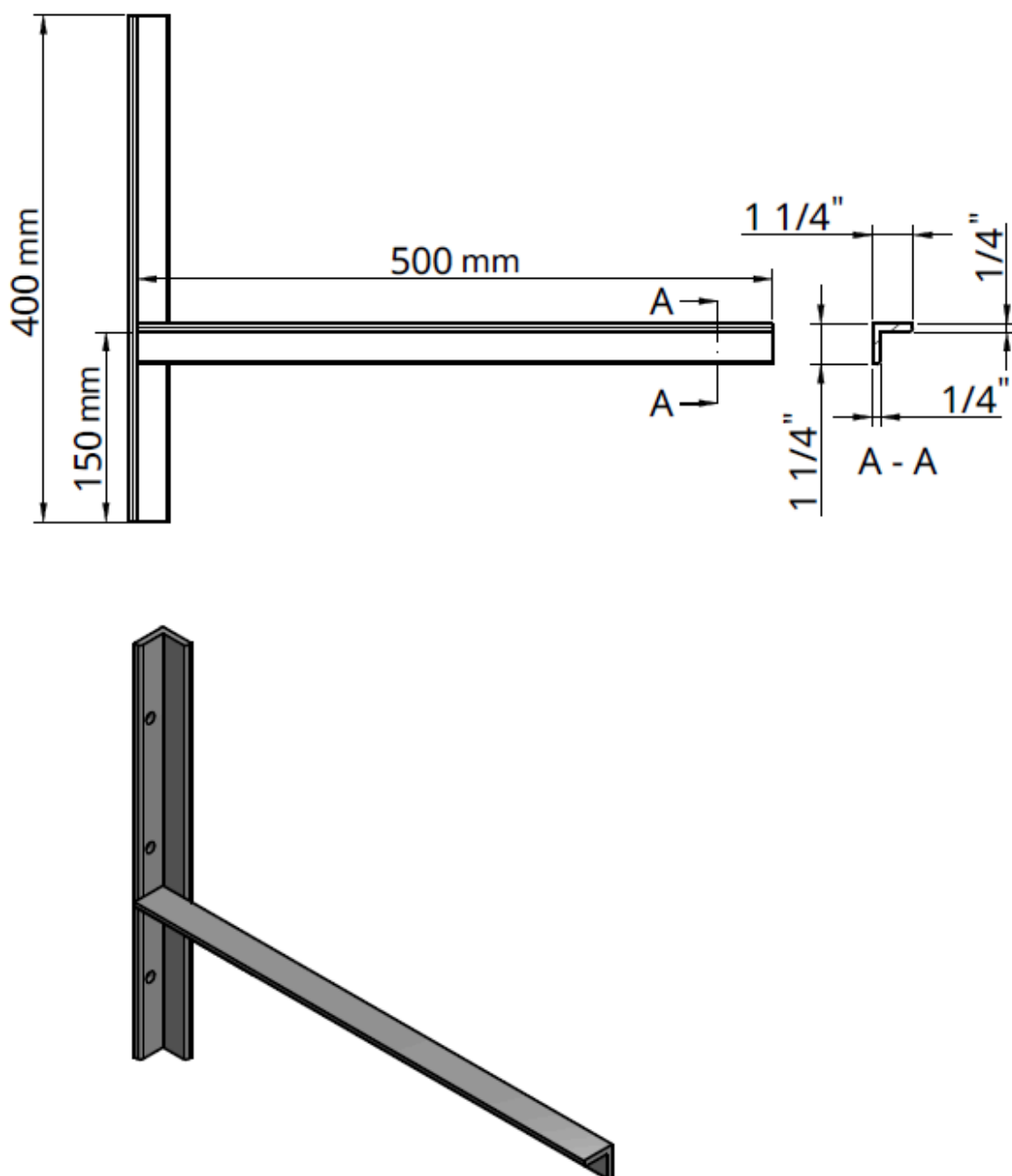
Figura 2 - Desenho técnico da cantoneira/suportes C2, destinada a unidades condensadoras com capacidade na faixa de 18.000 a 24.000 BTU/h
