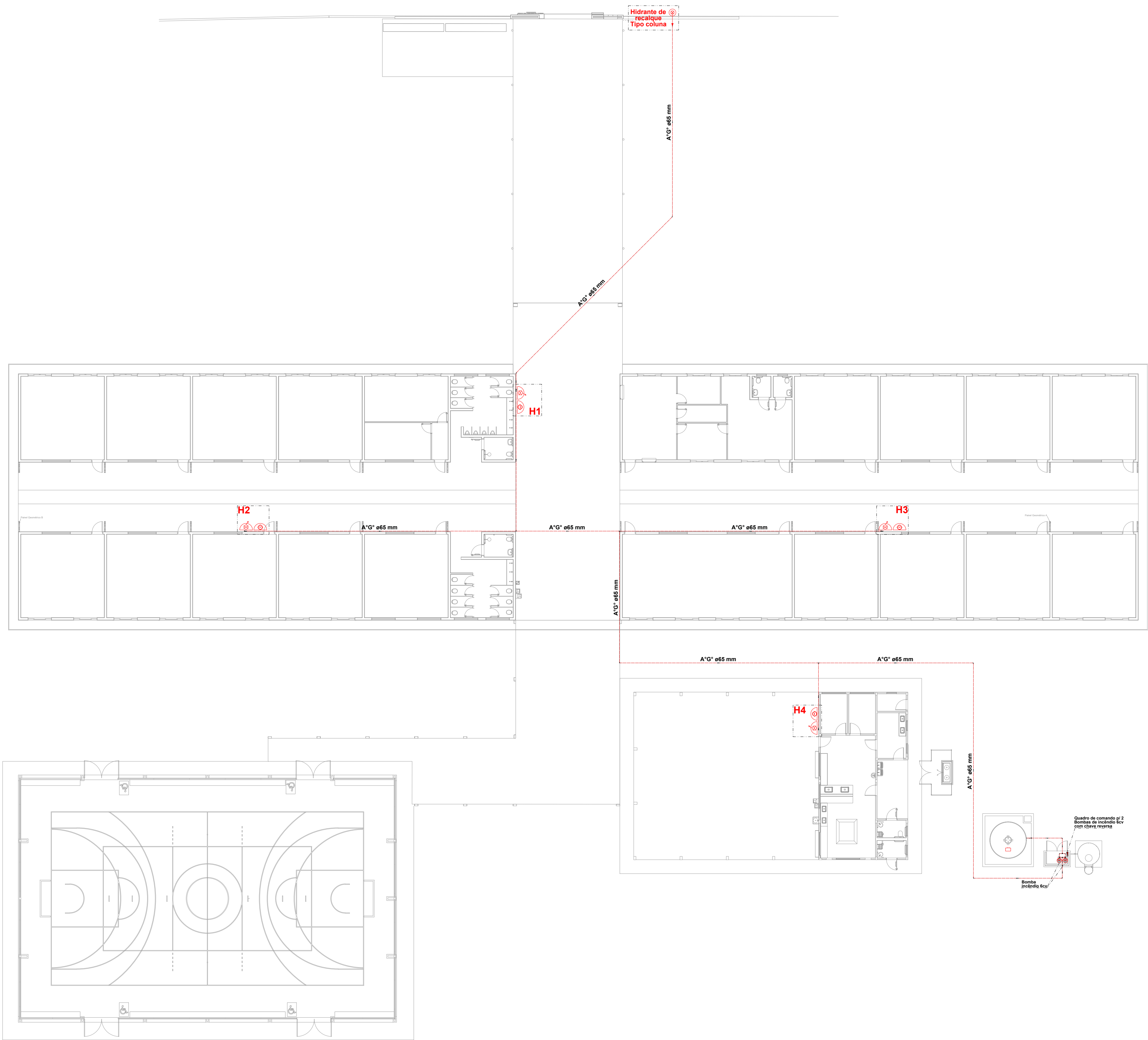
01 Planta baixa - Rede de hidrantes Escala: 1:200
