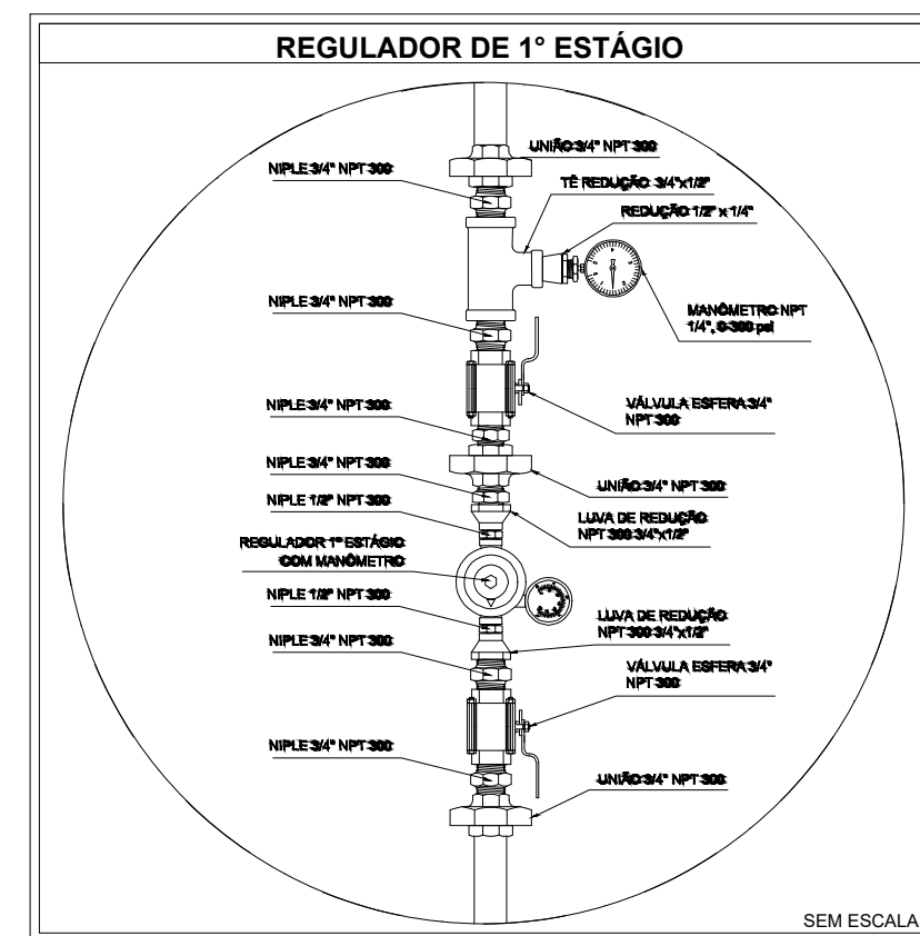
02 Detalhe "A" ESCALA: S/E
