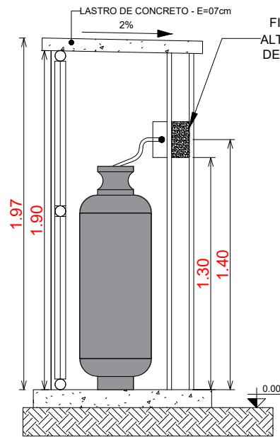
CORTE AA
