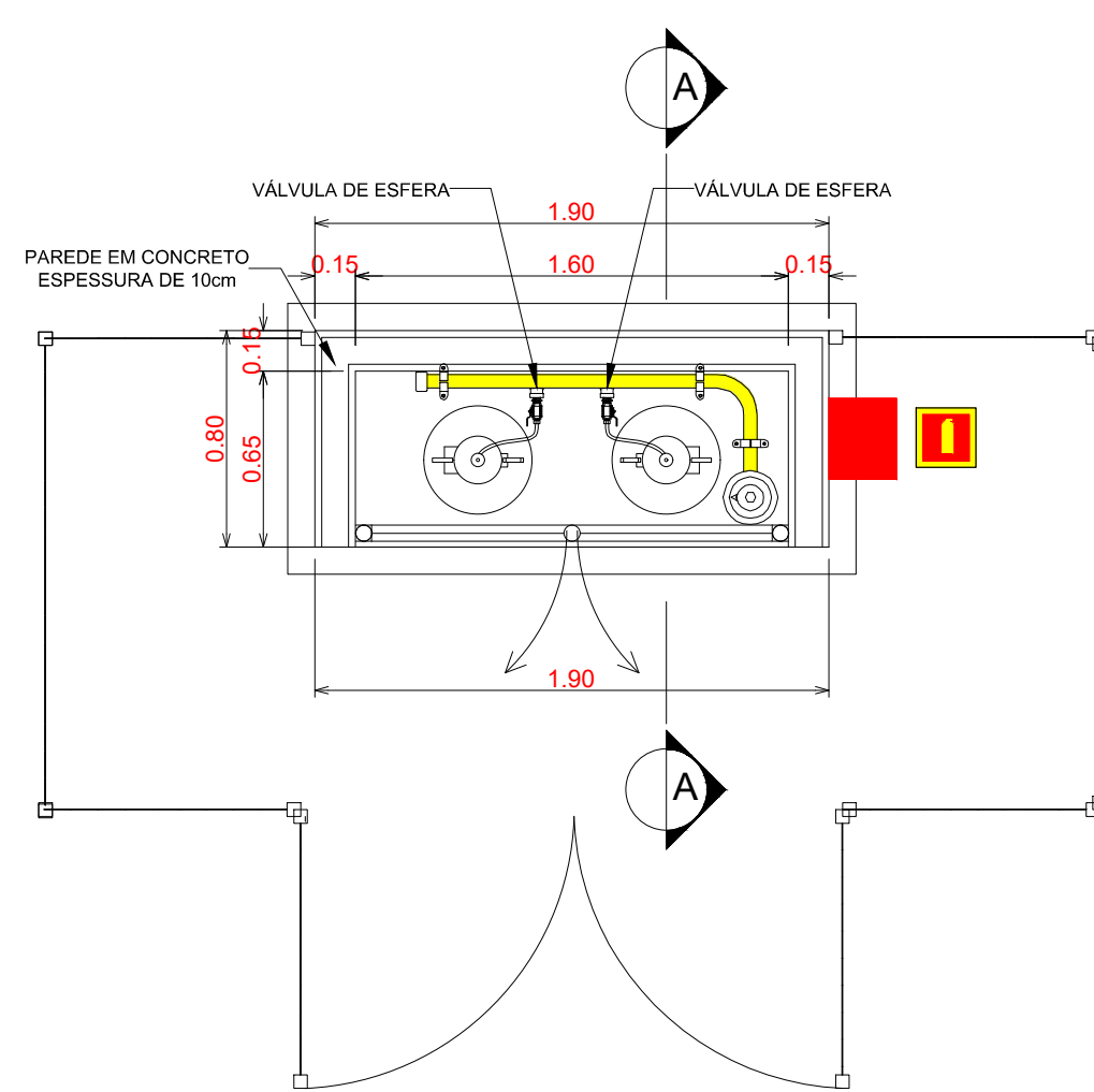
04 Detalhe central do GLP ESCALA: S/E
