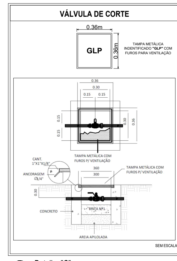
03 Detalhe "C" ESCALA: S/E
