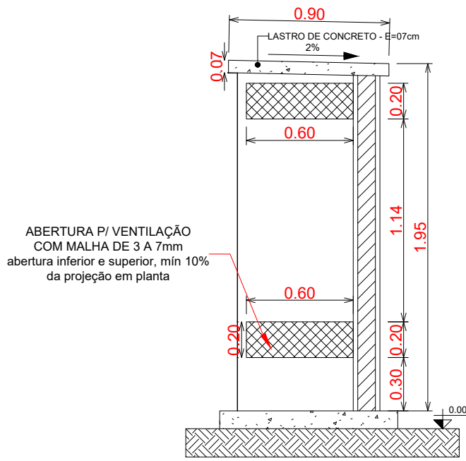
VISTA 1 VISTA LATERAL
