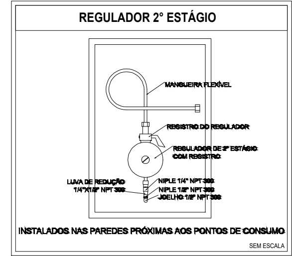
01 Detalhe "B" ESCALA: S/E
