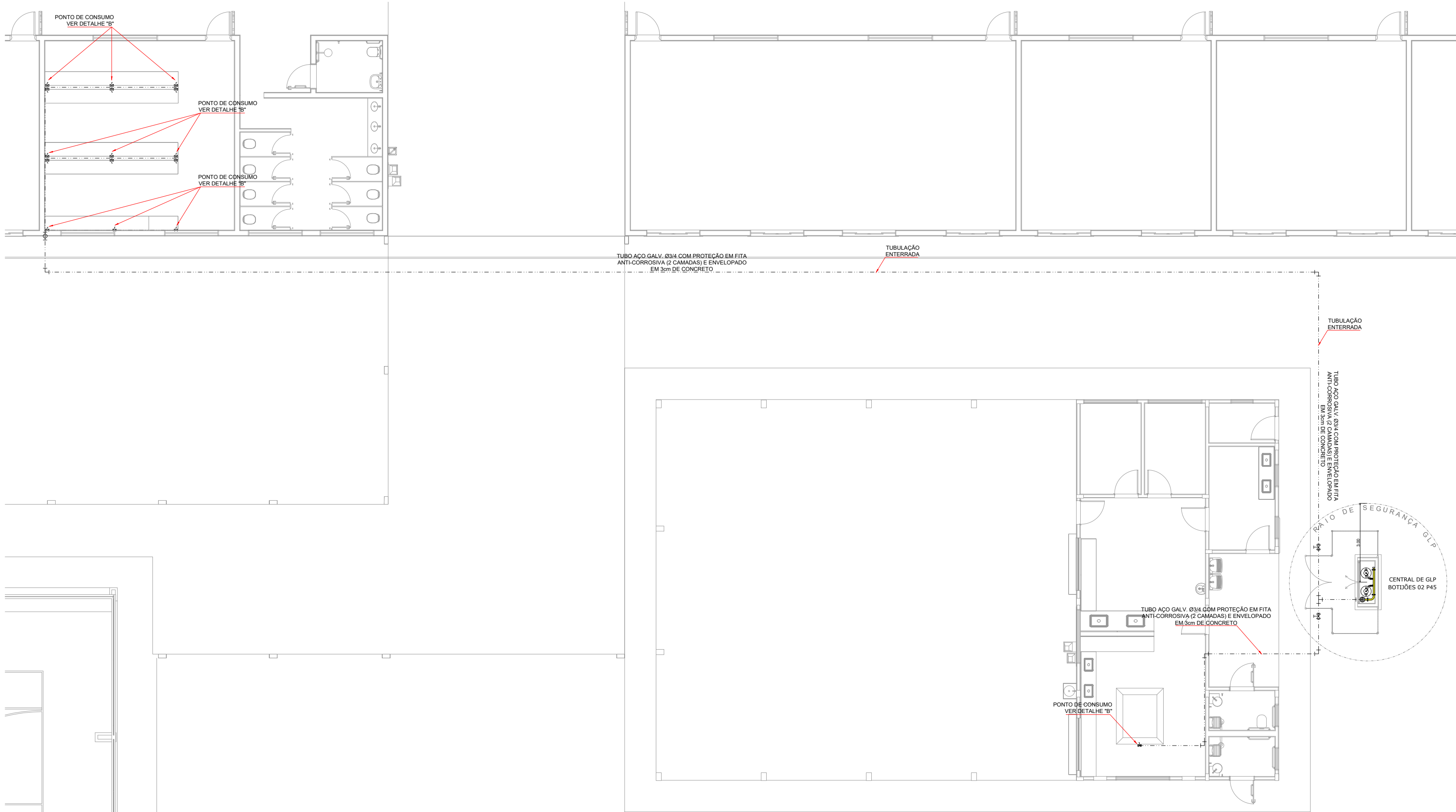
06 Planta baixa - Sistema de exaustão GLP ESCALA: 1:125
