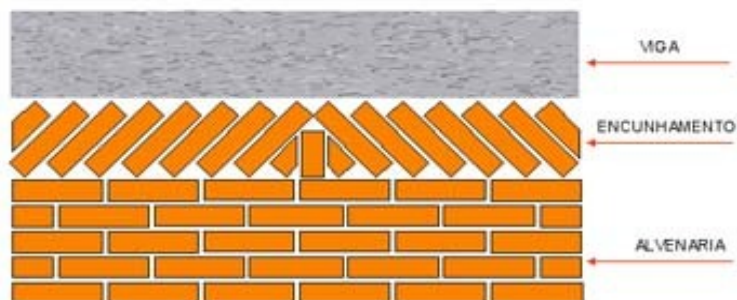
Encunhamento com tijolo cerâmico. Imagem ilustrativa.
