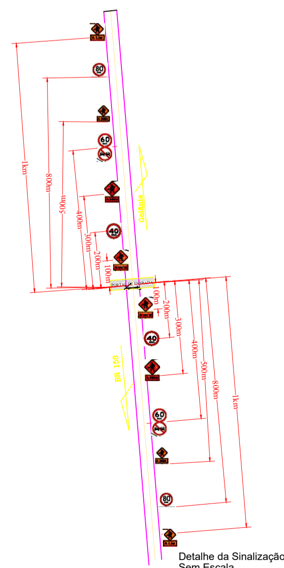
PLANTA DE SINALIZAÇÃO DE SEGURANÇA
