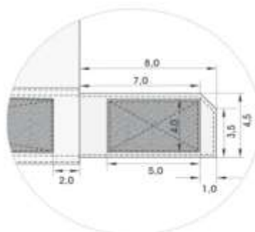
Detalhes da aba de ajuste do punho
