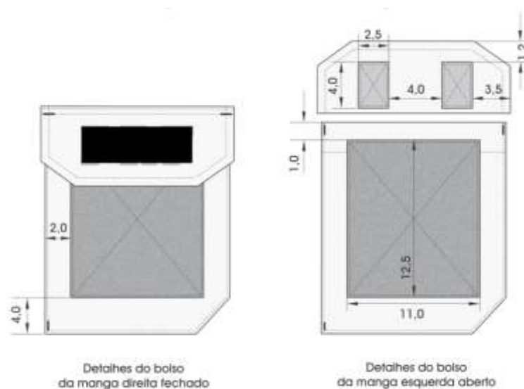
Figura 14 - Medidas e localização dos fechos de contatos dos bolsos nas mangas
