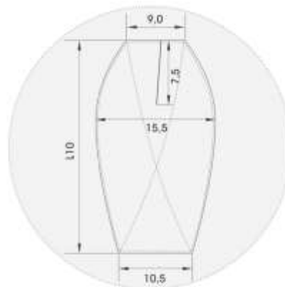
Figura 11 - Detalhes do reforço do cotovelo
