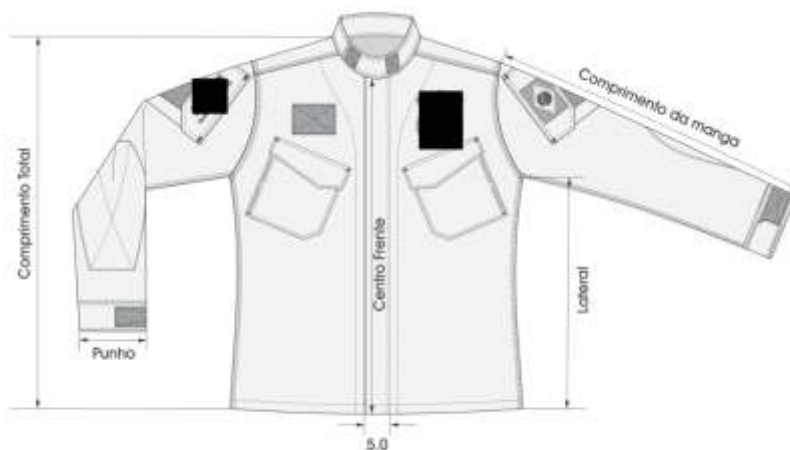
Figura 2 - Vista da Frente
