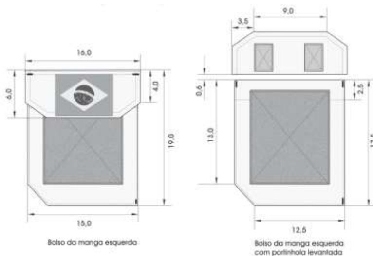
Figura 13 - Detalhes dos bolsos das mangas
