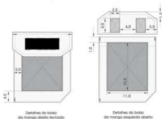
Figura 14 - Medidas e localização das fechos de contatos dos bolsos nas mangas
