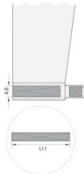
Figura 12 - Detalhes do punho
