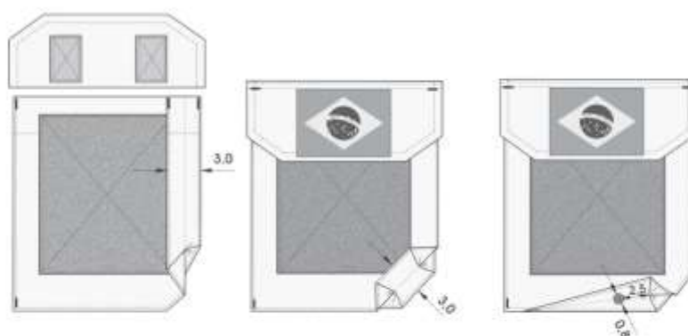
Figura 16 - Detalhes do fole dos bolsos (foles levantados)
