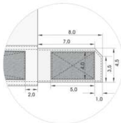
Detalhes da aleta de ajuste do punho
