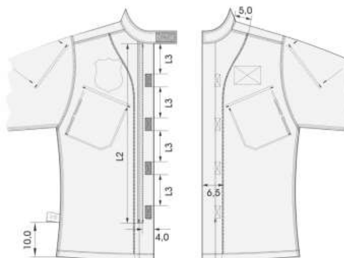
Figura 6 - Vista interna das frentes esquerda e direita
