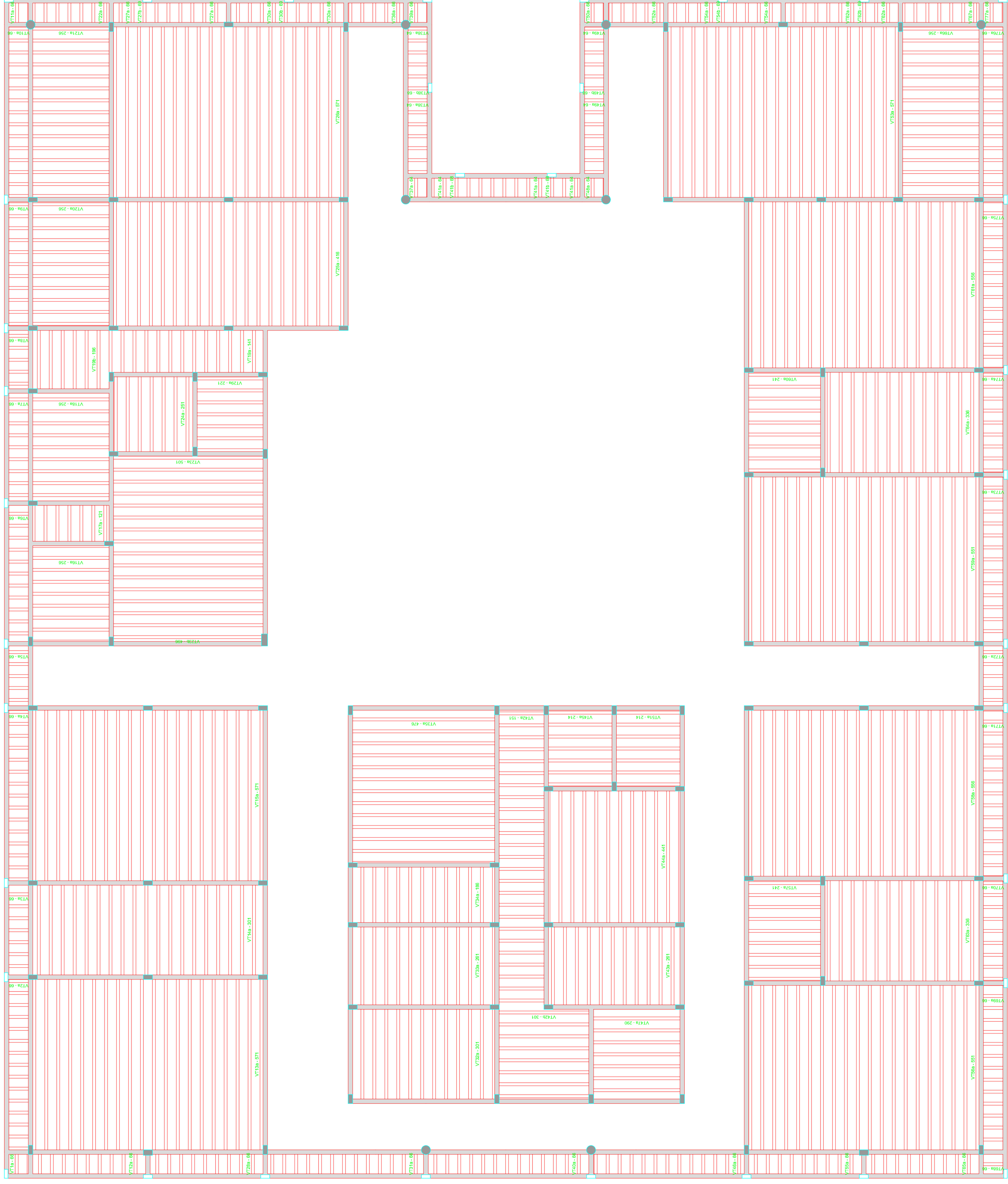
PLANTA DE VIGOTAS PRÉ-MOLDADAS Escala 1:50
