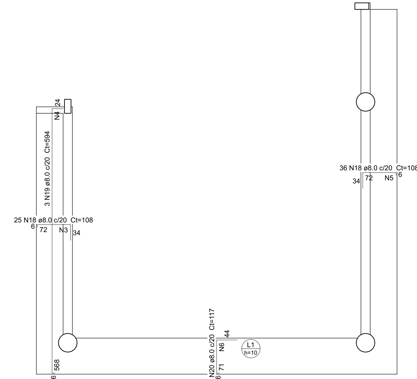
Armação negativa da laje - L1- COBERTURA escala 1:50
