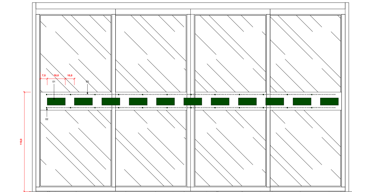
VISTA PORTA PORTAS AUTOMÁTICAS esc 1 : 20
