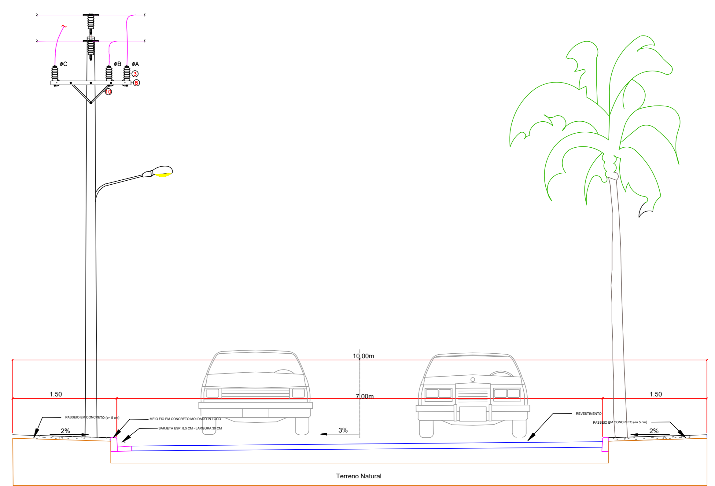
CORTE TRANSVERSAL DAS VIAS SEM ESCALA
