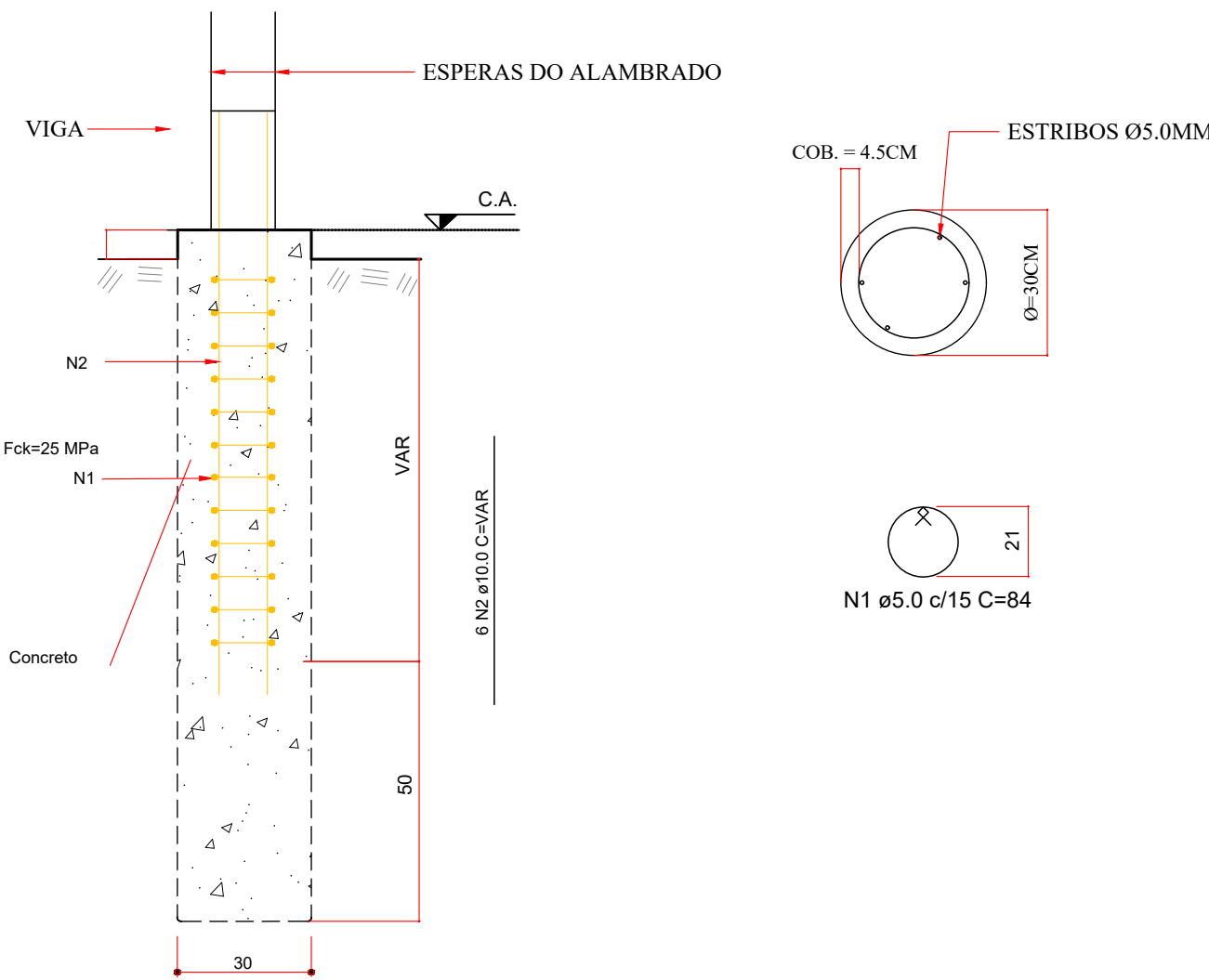
DETALHE DAS ESTACAS sem escala
