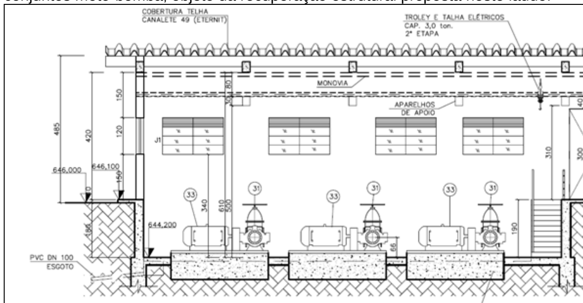
Figura 1. Corte esquemático da casa de bombas e das bases de concreto dos conjuntos moto-bomba, objeto da recuperação estrutural proposta neste laudo.
