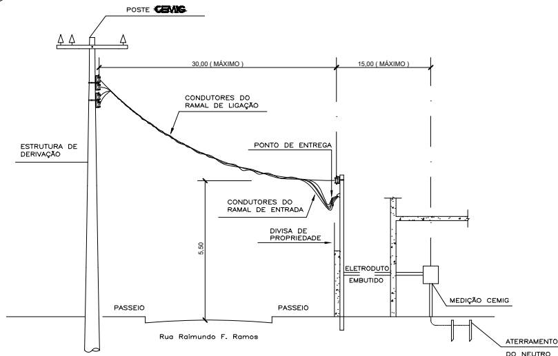
RAMAL DE LIGAÇÃO SESCALA OBS: MEDIDAS EM METROS
