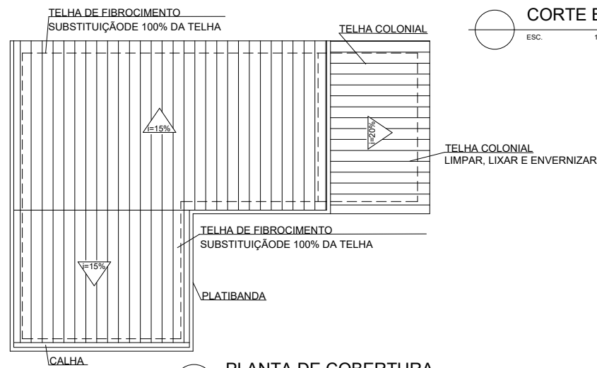
PLANTA DE COBERTURA ESC. 1:100 COBERTURA FIBROCIMENTO 130,29 m² COBERTURA CERÂMICA 32,08 m²
