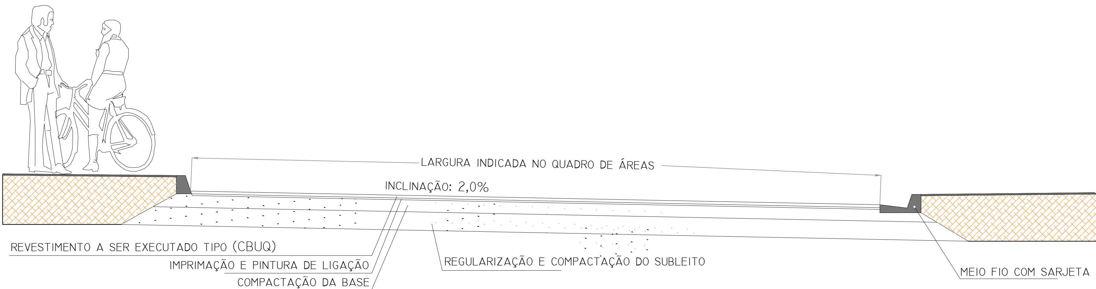
Corte da Seção Transversal Sem Escala
