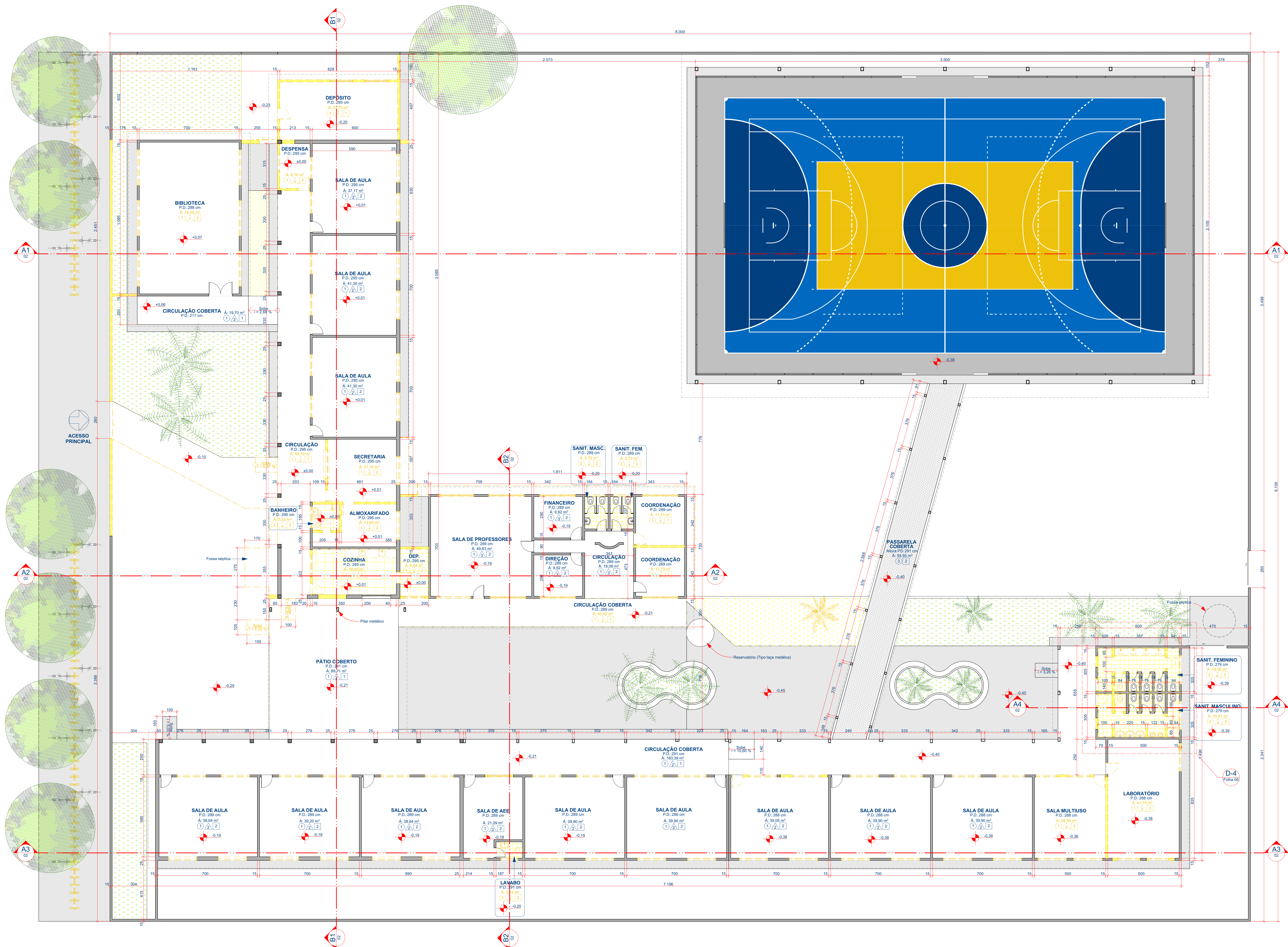
09 PLANTA DE DEMOLIÇÕES Escala: 1:100
