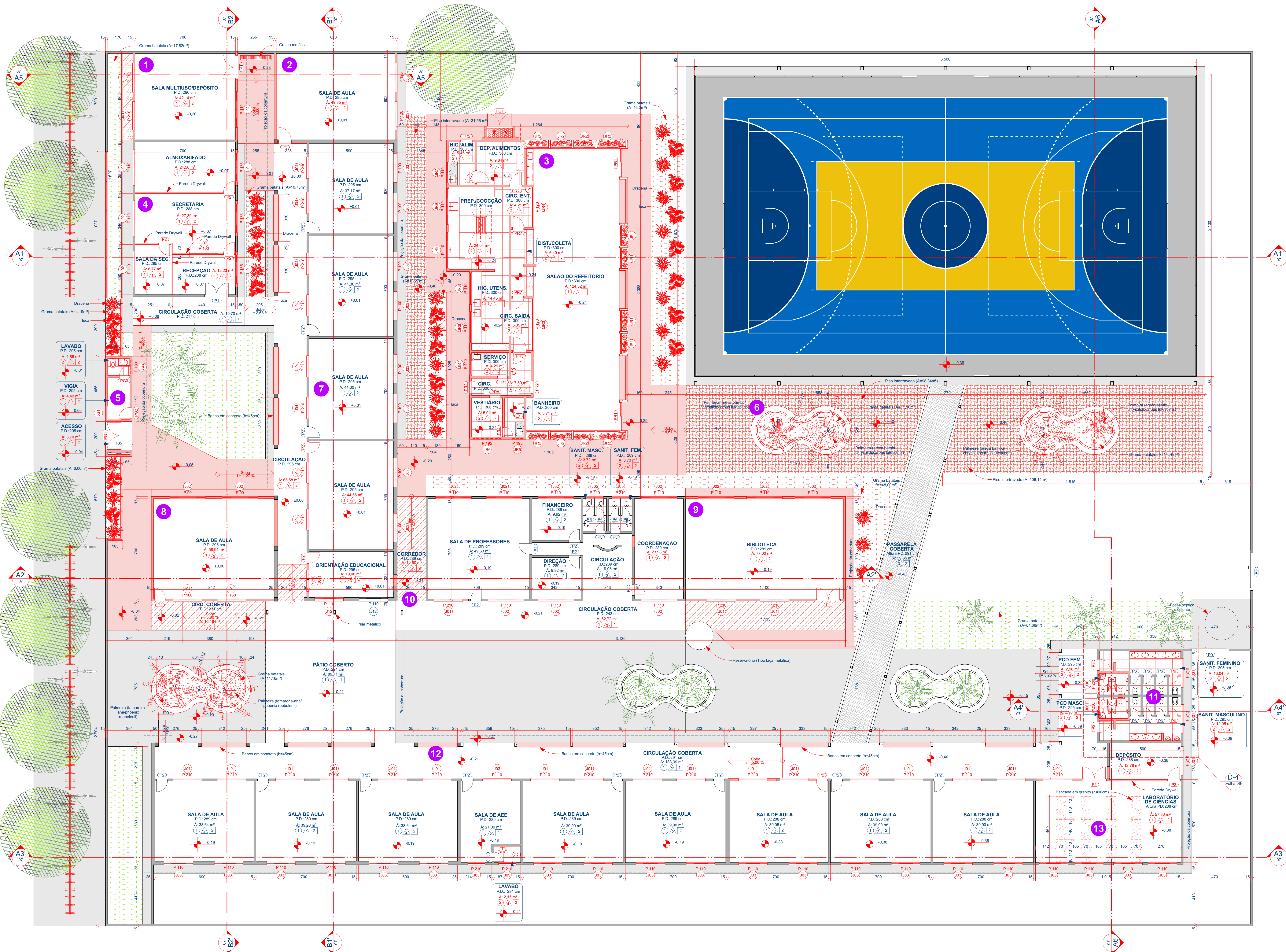
10 PLANTA DE CONSTRUÇÕES Escala: 1:100
