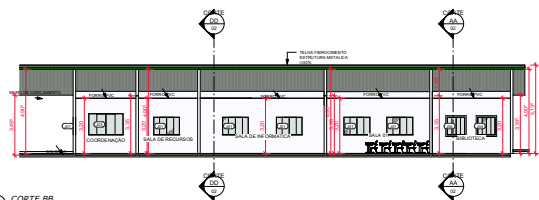
2 CORTE BB 1:200
