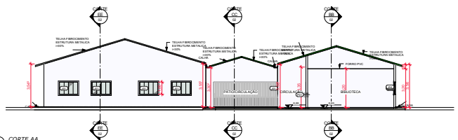
1 CORTE AA 1:200
