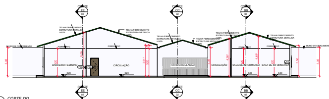
4 CORTE DD 1:200
