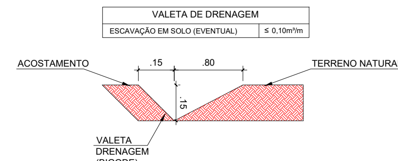
Seção Transversal - Etapa 3 Esc.H.: 1/50
