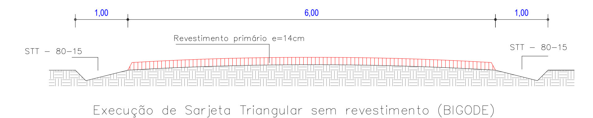
Sarjeta triangular sem revestimento - STT 80-15
