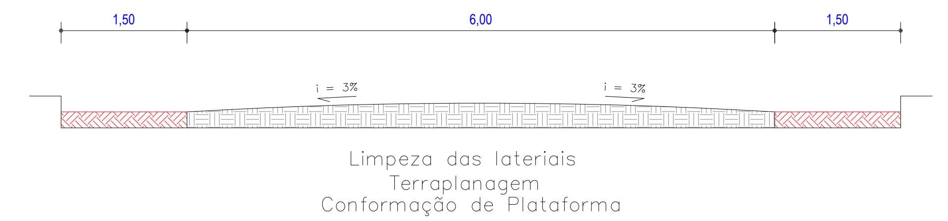
Seção Transversal Típica - Etapa 1 Esc.H.: 1/50
