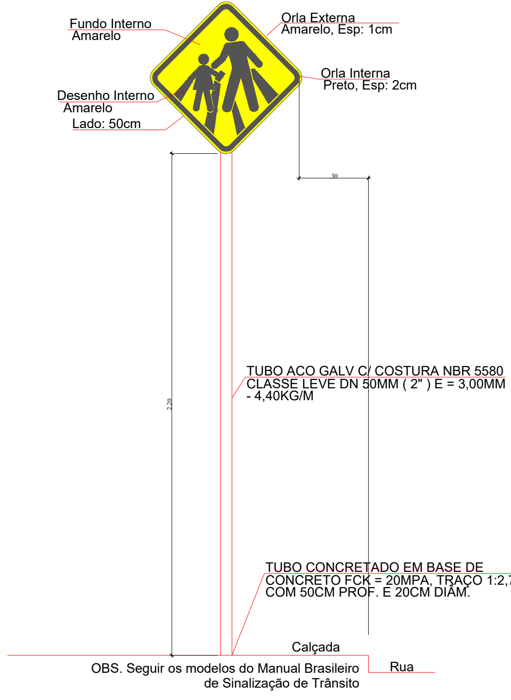
DETALHE PLACA FAIXA DE PEDESTRES A-33b
