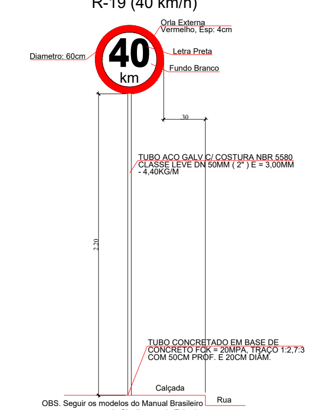
DETALHE PLACA VELOCIDADE MÁXIMA R-19 (40 km/h)
