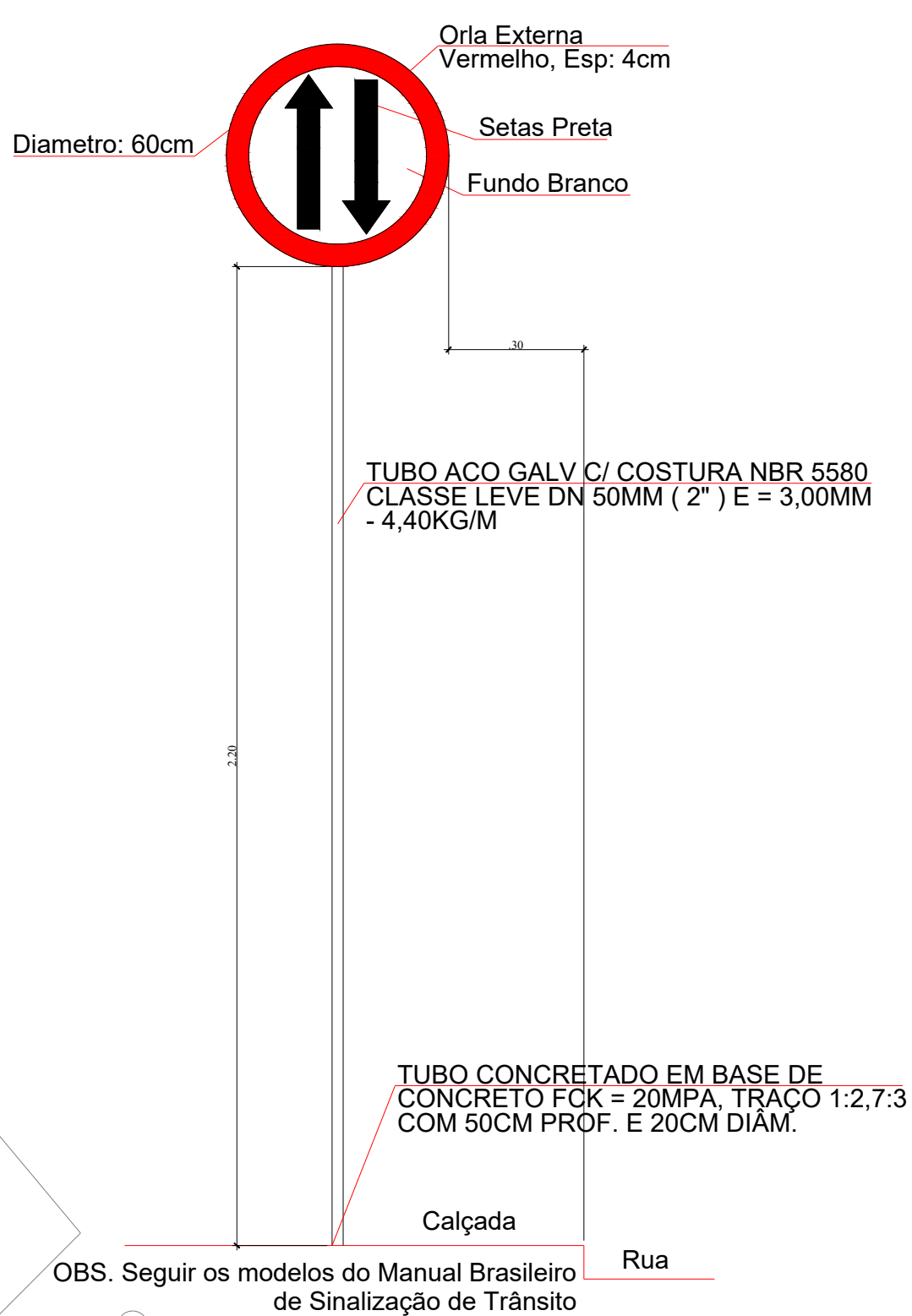
DETALHE PLACA DUPLO SENTIDO DE CIRCULAÇÃO R-28
