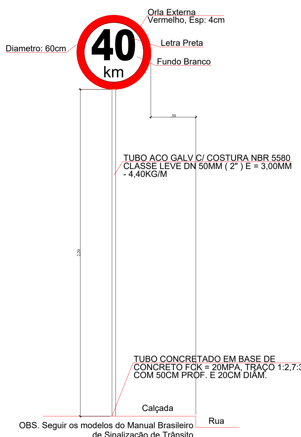
DETALHE PLACA VELOCIDADE MÁXIMA R-19 (40 km/h)
