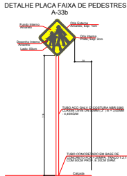
DETALHE PLACA FAIXA DE PEDESTRES A-33b
