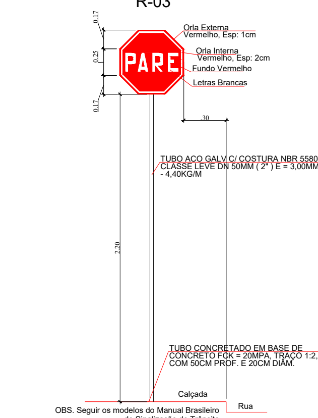
DETALHE PLACA SENTIDO PROIBIDO R-03
