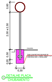
DETALHE PLACA FAIXA DE PEDESTRES A-33b
