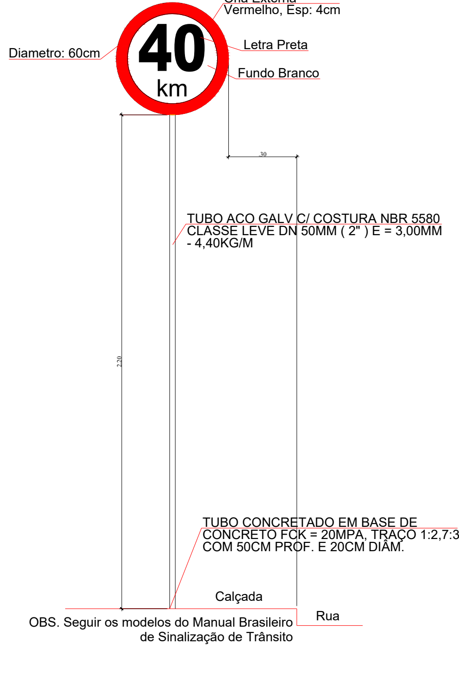
DETALHE PLACA VELOCIDADE MÁXIMA R-19 (40 km/h)
