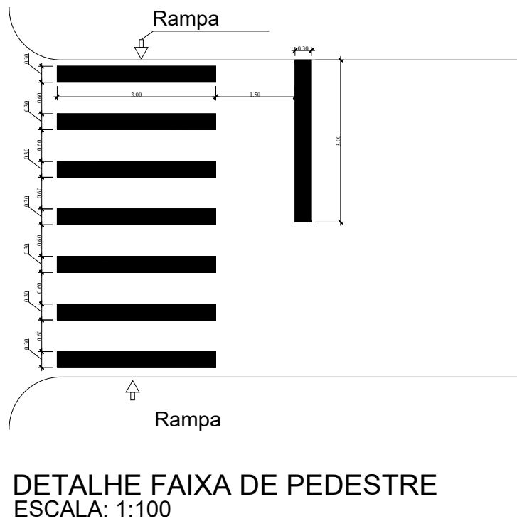
DETALHE FAIXA DE PEDESTRE ESCALA: 1:100
