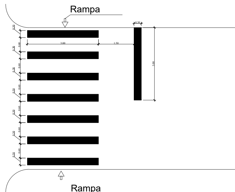
DETALHE FAIXA DE PEDESTRE ESCALA: 1:100
