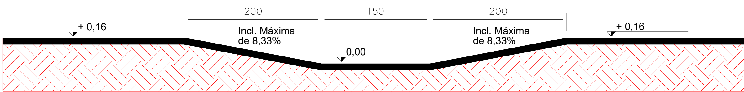
Cortes em detalhes Rebaixamento da calçada
