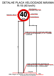
DETALHE PLACA VELOCIDADE MÁXIMA R-19 (40 km/h)
