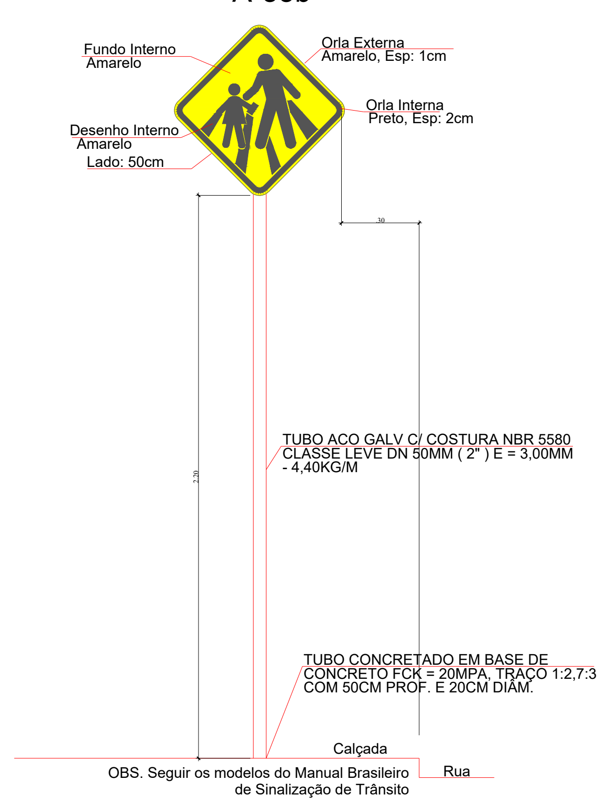
DETALHE PLACA FAIXA DE PEDESTRES A-33b
