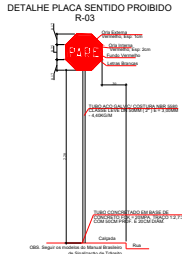
DETALHE PLACA SENTIDO PROIBIDO R-03
