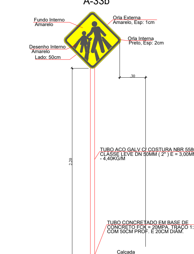
DETALHE PLACA FAIXA DE PEDESTRES A-33b
