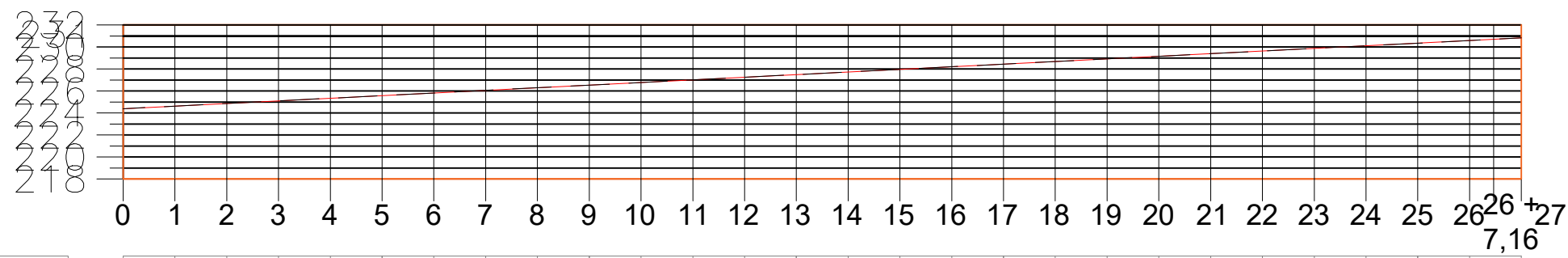
Perfil - TRECHO 05 - AV. AIRTON SENNA
