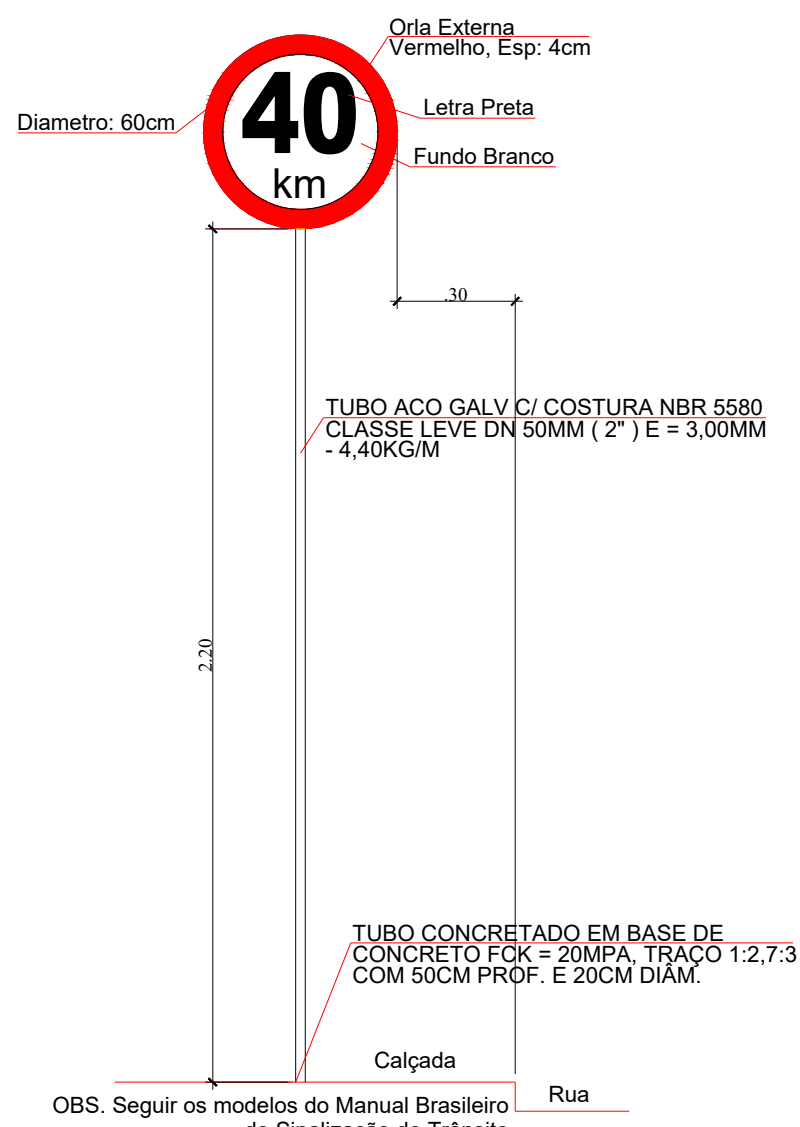
DETALHE PLACA VELOCIDADE MÁXIMA R-19 (40 km/h)
