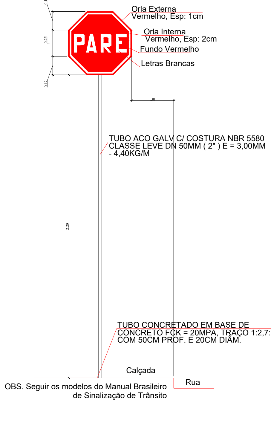
DETALHE PLACA SENTIDO PROIBIDO R-03
