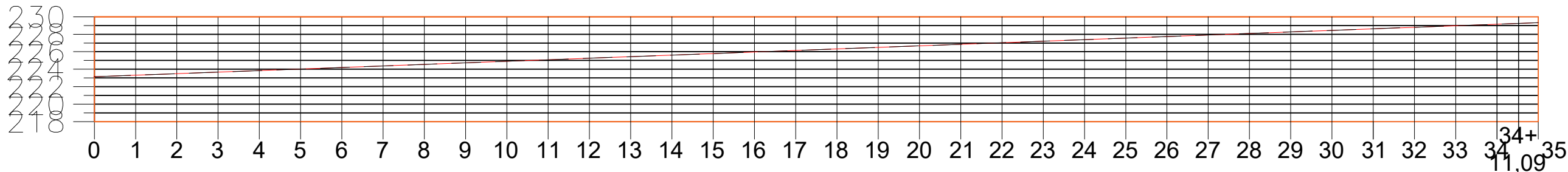
Perfil - TRECHO 06 - RUA MARIANO ARAÚJO LIMA
