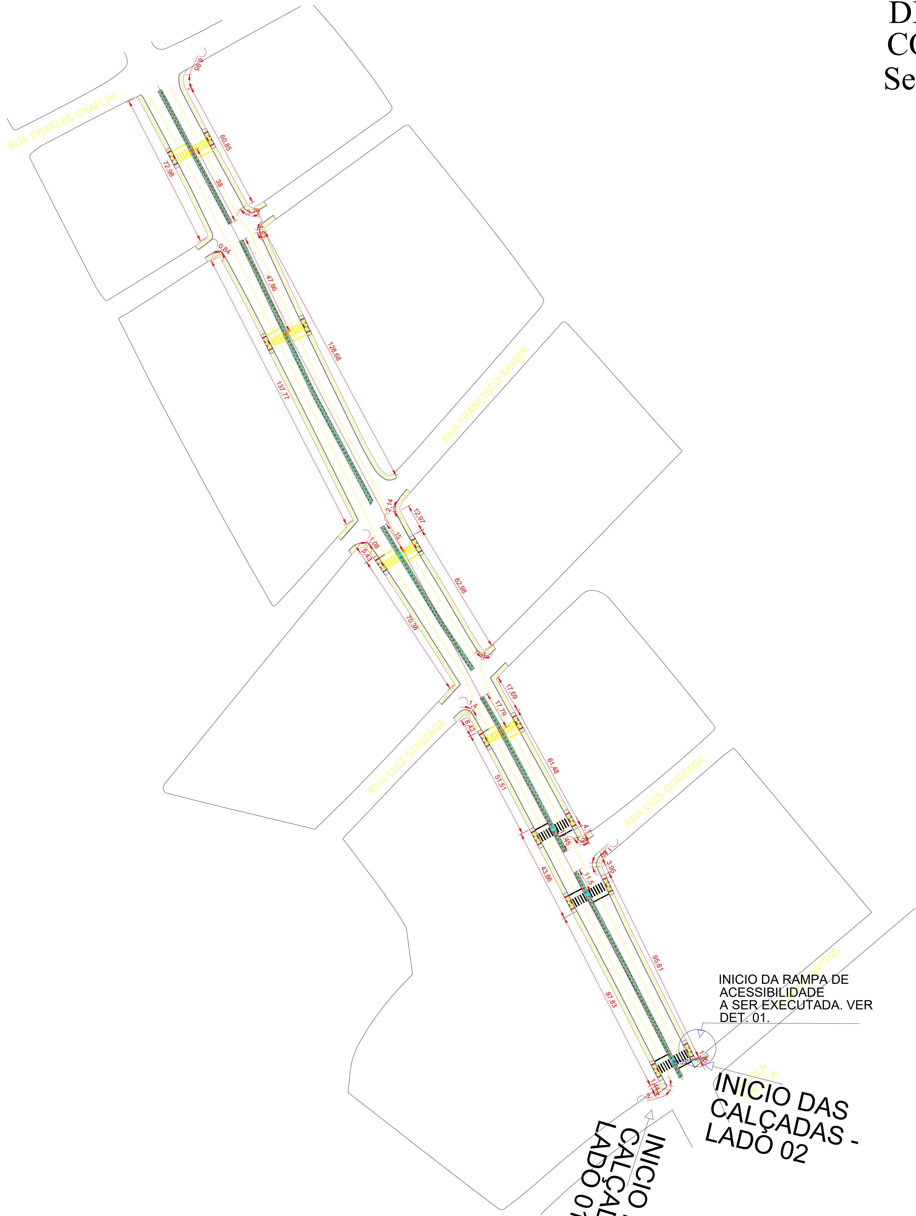
TRECHO 05 - AV. AYRTON SENNA ESCALA: 1:750
