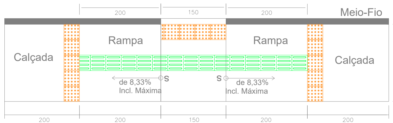
DET.01 - Detalhes do Calçamento Rampas e Juntas de Dilatação
