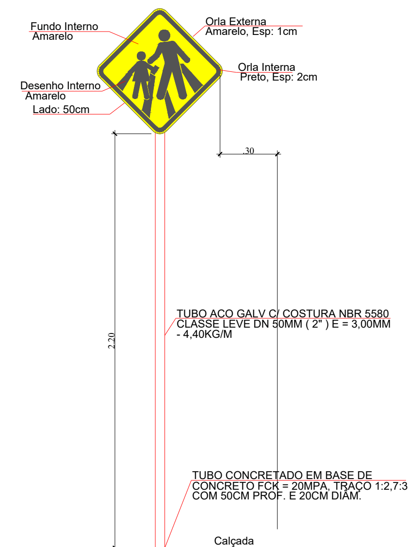
DETALHE PLACA FAIXA DE PEDESTRES A-33b
