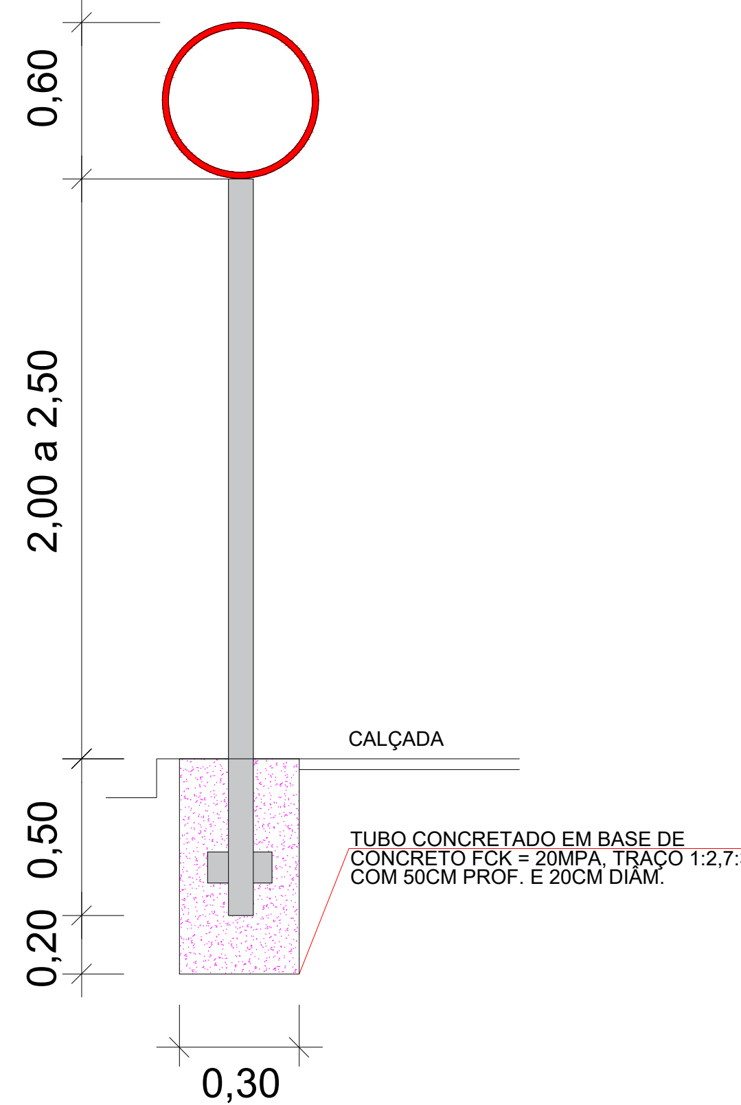
DETALHE PLACA CHUBAMENTO
