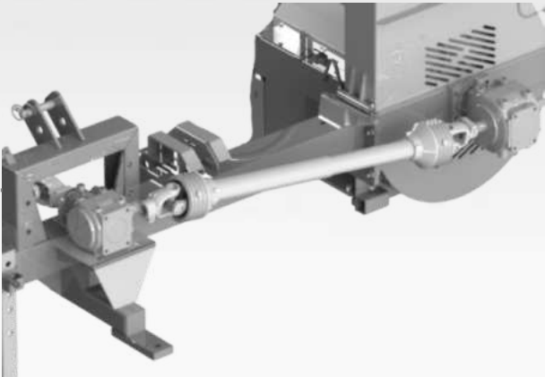
CUSTOM 950 Transmissão feita através de caixa de transmissão e cardan.
