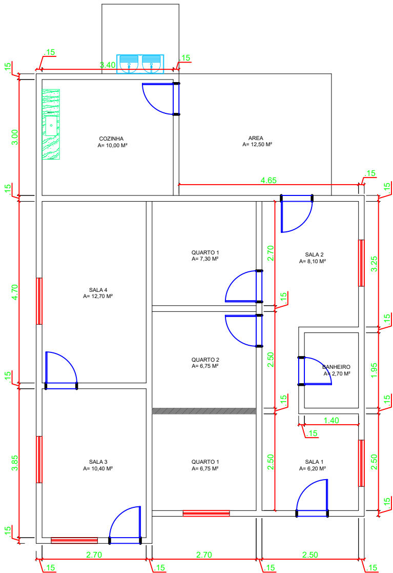
PLANTA BAIXA Area: 100,00 m²
