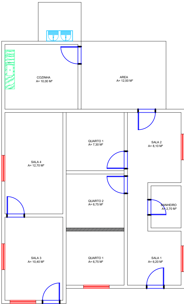
PLANTA BAIXA Area: 100,00 m²
