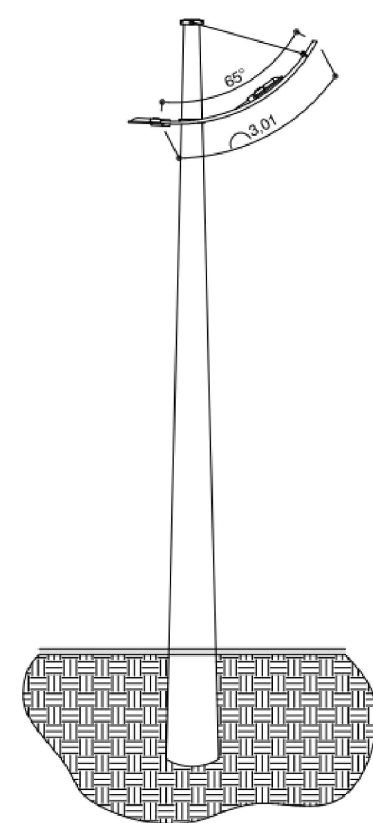
03 DETALHE - LUMINÁRIA PÚBLICA EM BRACÇO SEXTANTE SEM ESCALA
