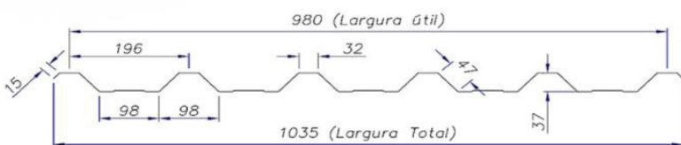
imagem telha metálica trapezoidal TP40-980
