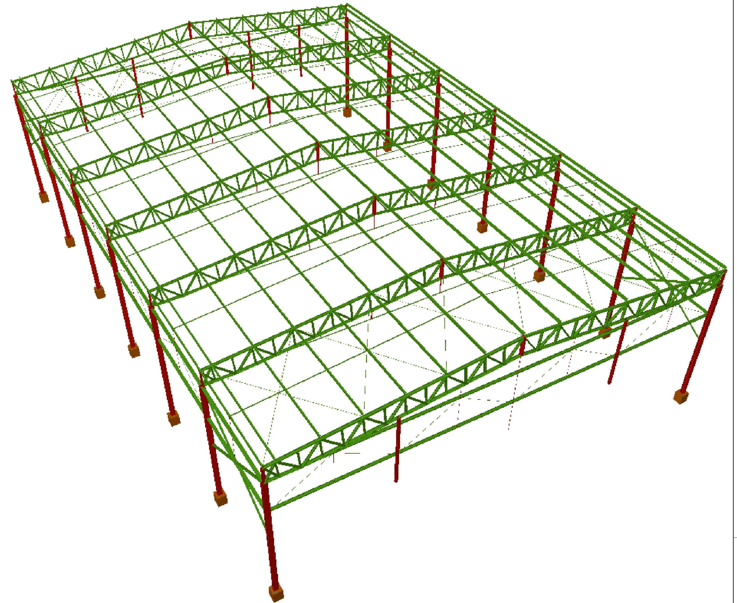
ISOMETRIA DA ESTRUTURA ESC.1:50
