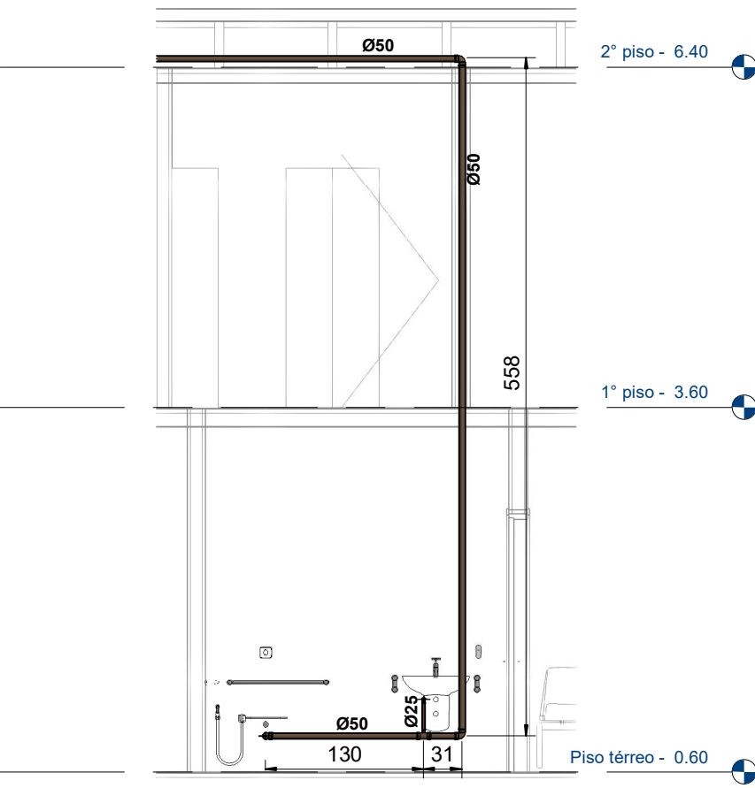
Section 1 1 : 50
