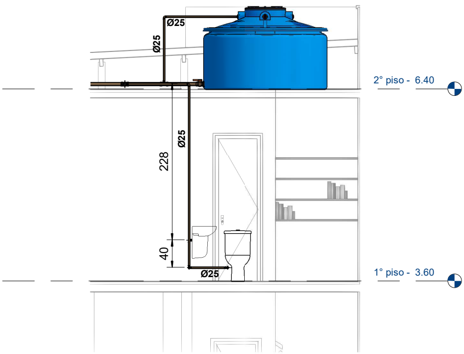
Section 5 1 : 50
