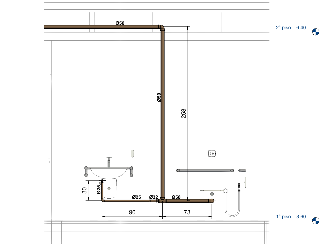
Section 4 1 : 25
