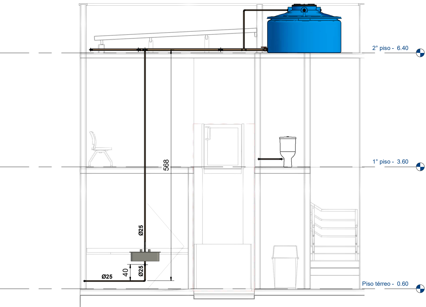
Section 3 1 : 50
