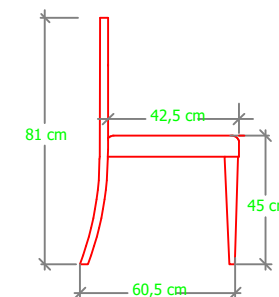
VISTAS
