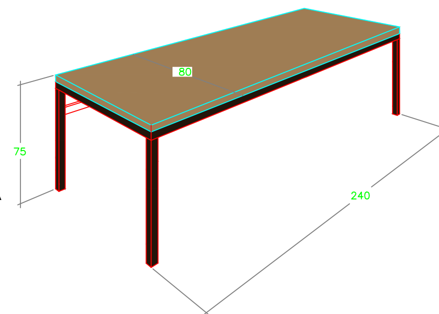
PERSPECTIVA MESA
