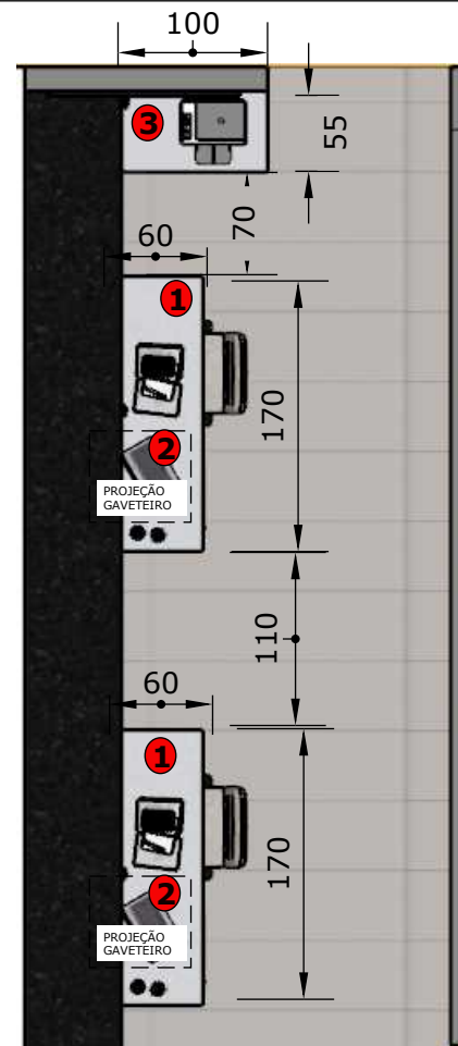
PLANTA BAIXA
