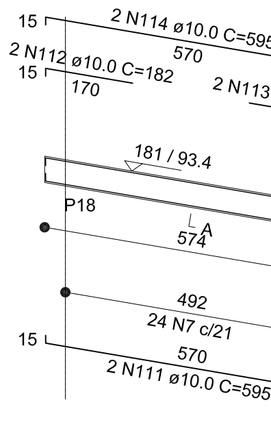
V39 (20 x 50)
