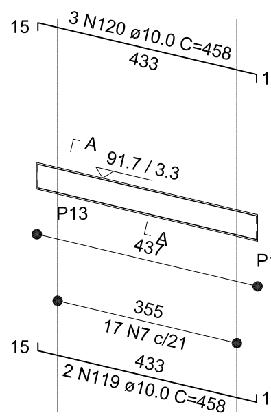
V42 (20 x 50)
