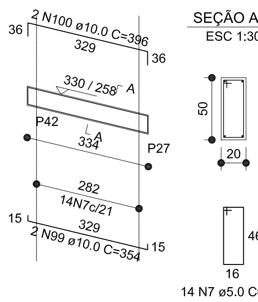
V41 (20 x 50)
