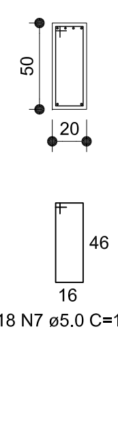
SEÇÃO A-A
