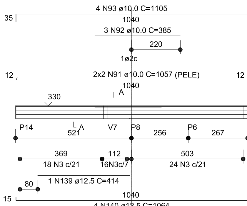
V29 (20 x 60)
