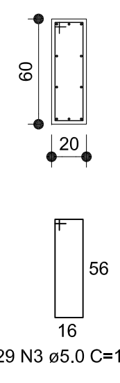
SEÇÃO A-A
