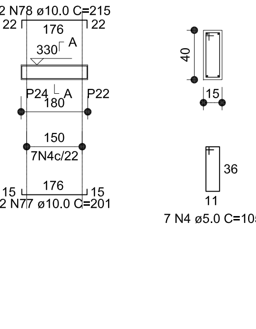
V23 (15 x 40)
