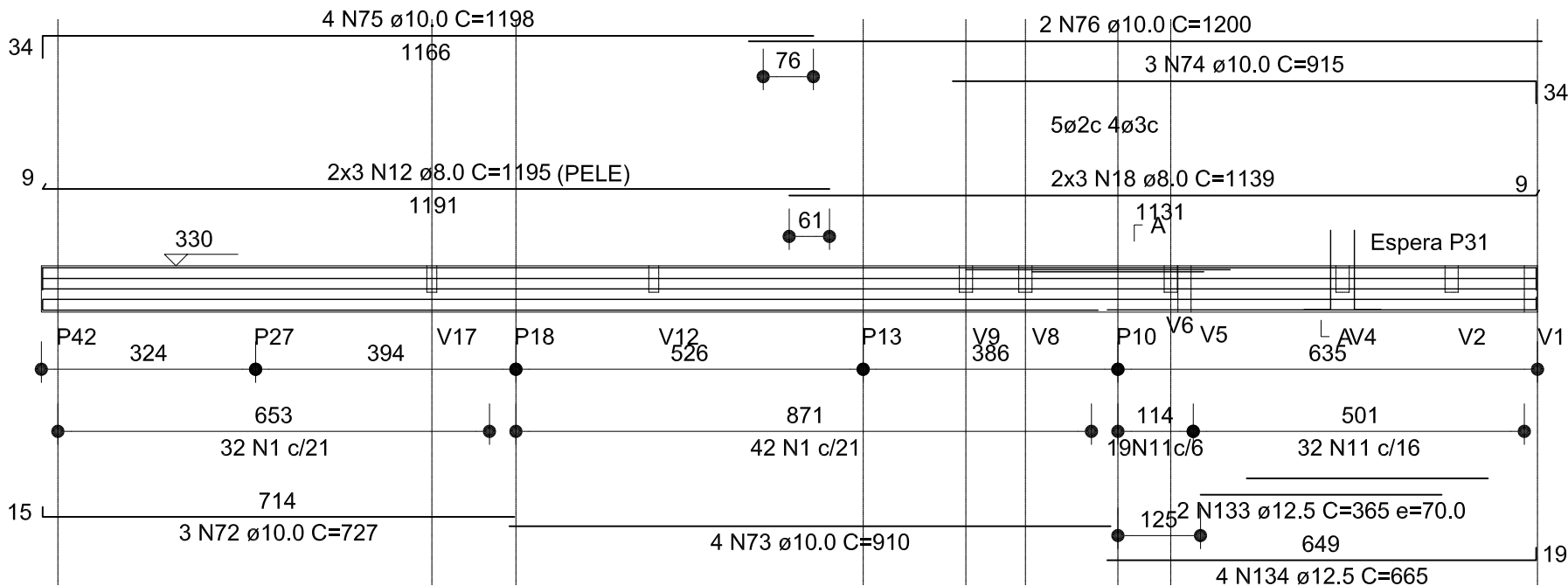
V22 (20 x 70)
