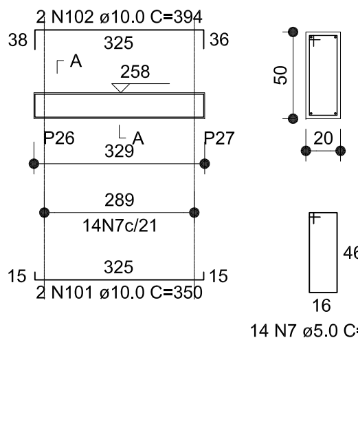
SEÇÃO A-A
