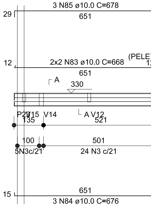
V26 (20 x 60)
