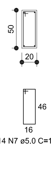
SEÇÃO A-A
