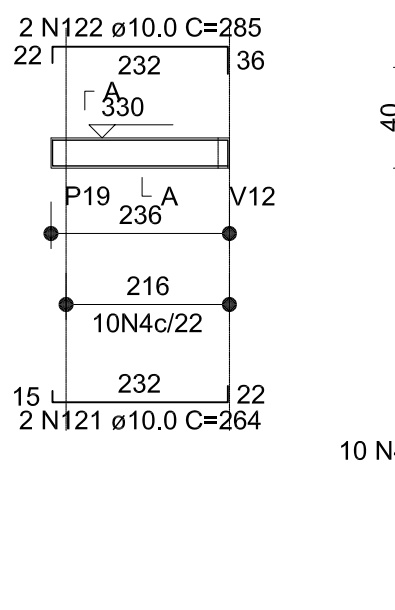
V43 (15 x 40)
