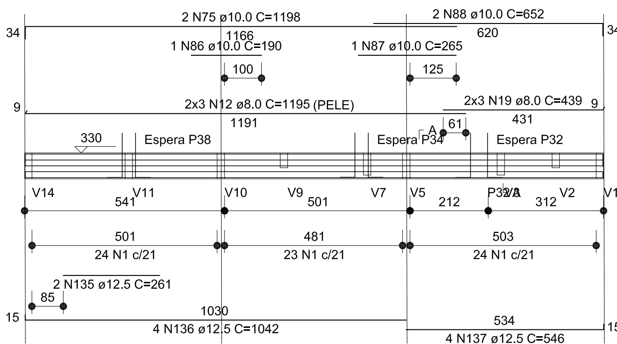
V27 (20 x 70)
