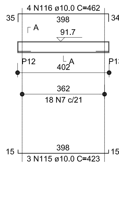
V40 (20 x 50)
