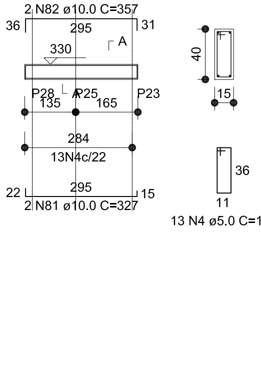
SEÇÃO A-A
