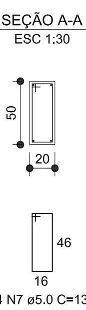
V41 (20 x 50)
