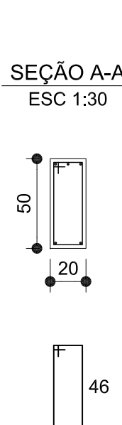
SEÇÃO A-A
