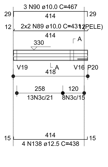
V28 (20 x 60)
