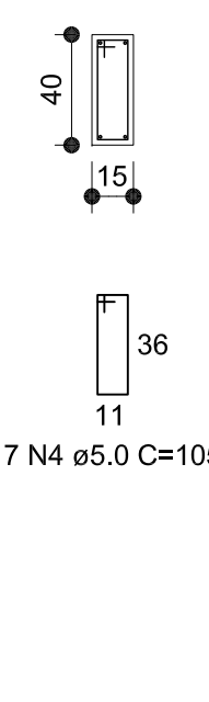
SEÇÃO A-A
