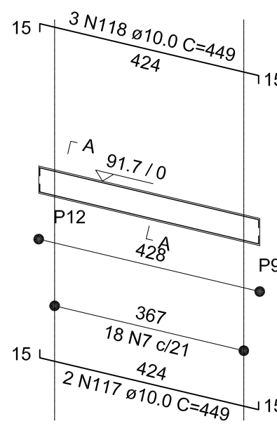
V41 (20 x 50)
