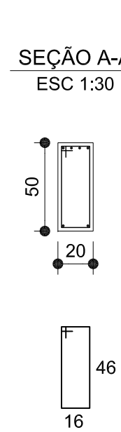
SEÇÃO A-A
