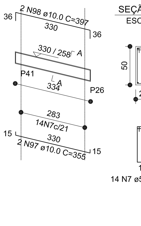
V32 (20 x 50)
