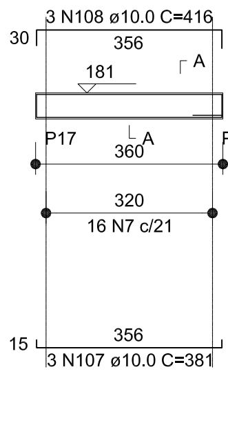
V37 (20 x 50)
