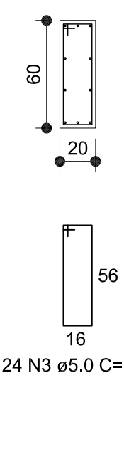
SEÇÃO A-A
