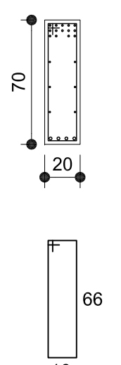
SEÇÃO A-A
