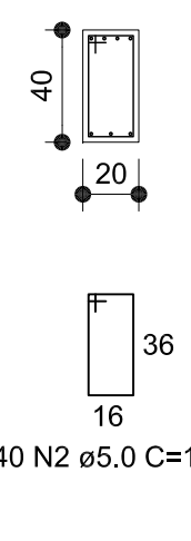
SEÇÃO A-A
