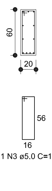
SEÇÃO A-A
