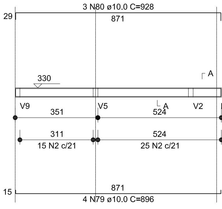
V24 (20 x 40)
