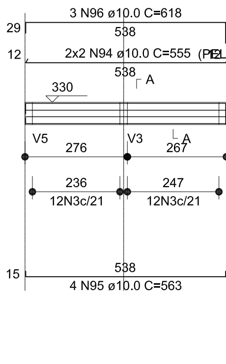
V30 (20 x 60)
