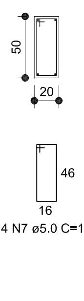
V42 (20 x 50)
