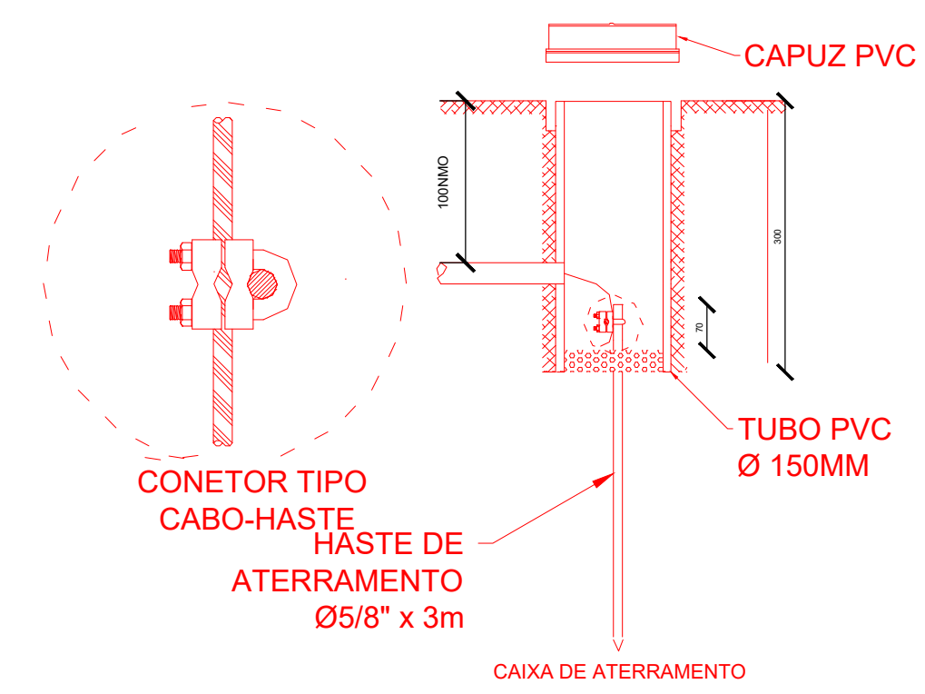
4 DETALHE CX. DE ATERRAMENTO SEM ESCALA
