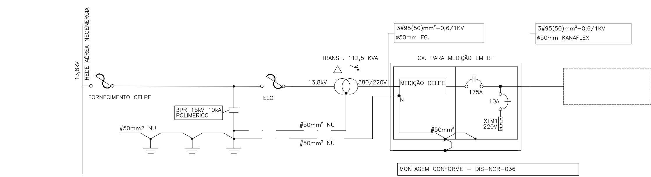
5 SE 112,5 kVA - DIAGRAMA UNIFILAR SEM ESCALA
