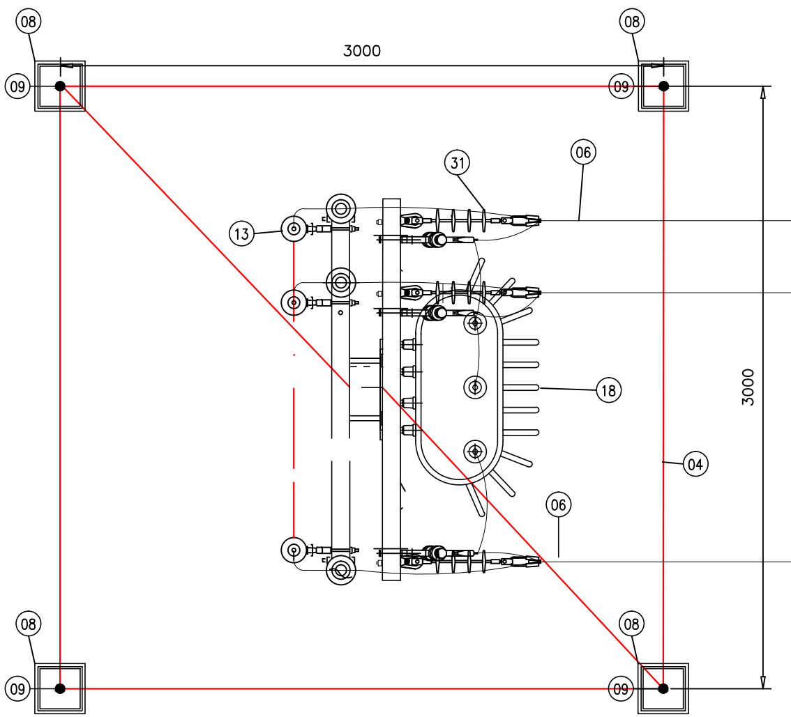
3 SE 112,5 kVA - VISTA SUPERIOR SEM ESCALA
