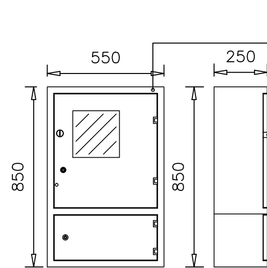
5 DETALHE CX. DE MEDIÇÃO EM BT SEM TC'S PADRÃO CELPE USO EXTERNO SEM ESCALA
