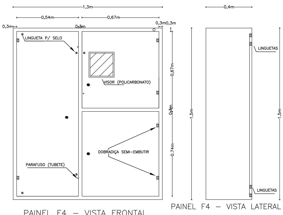
4 DETALHE CX. DE MEDIÇÃO F4 PADRÃO NEOENERGIA SEM ESCALA
