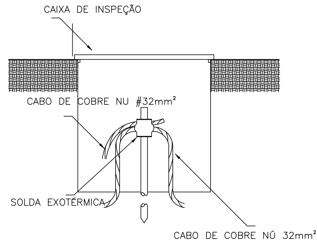
6 DETALHE CX. DE INSPEÇÃO SEM ESCALA
