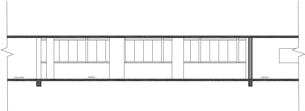
01 CORTE A 1/100
