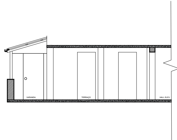
04 CORTE D 1/100
