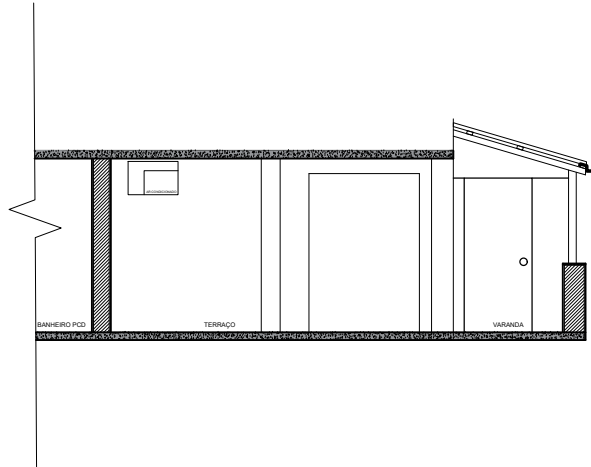
03 CORTE C 1/100
