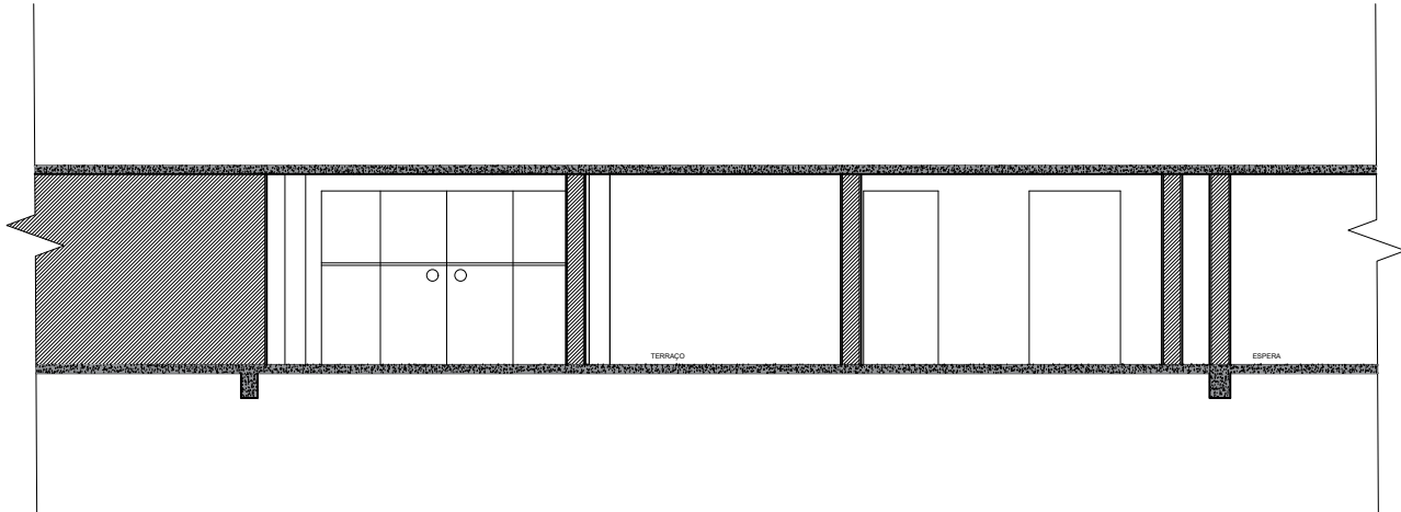
02 CORTE B 1/100
