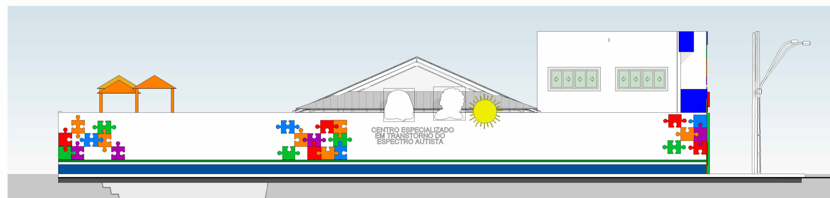
1 VISTA LATERAL 1 : 100
