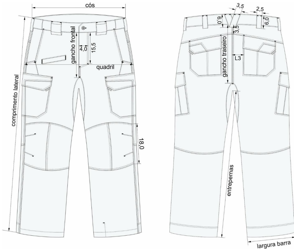
Figura 1 – Vistas frontal e traseira da calça
