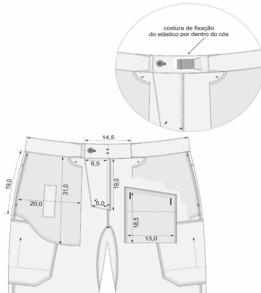
Figura 11 - Detalhes do pertingal e dos forros dos bolsos na frente da Calça
