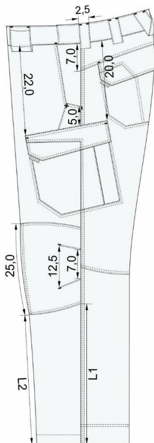
Figura 3 – Vista lateral da calça tática
