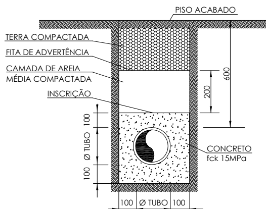
DETALHE DO ENVELOPAMENTO ($/ESCALA)
