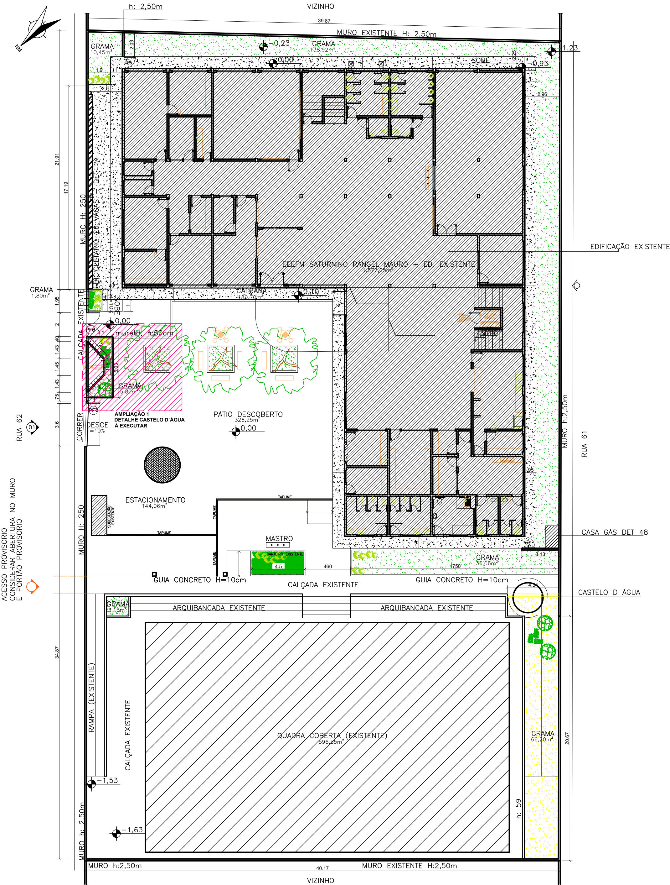
IMPLANTAÇÃO EXISTENTE ESC: 1/200
