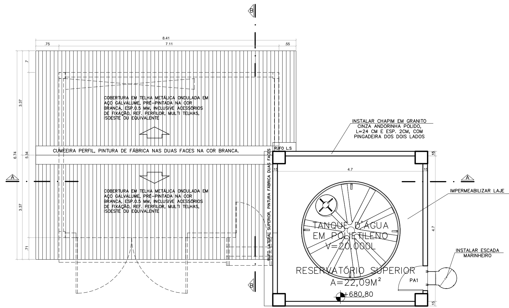
PLANTA BAIXA RESERVATÓRIO SUPERIOR ESC 1/50
