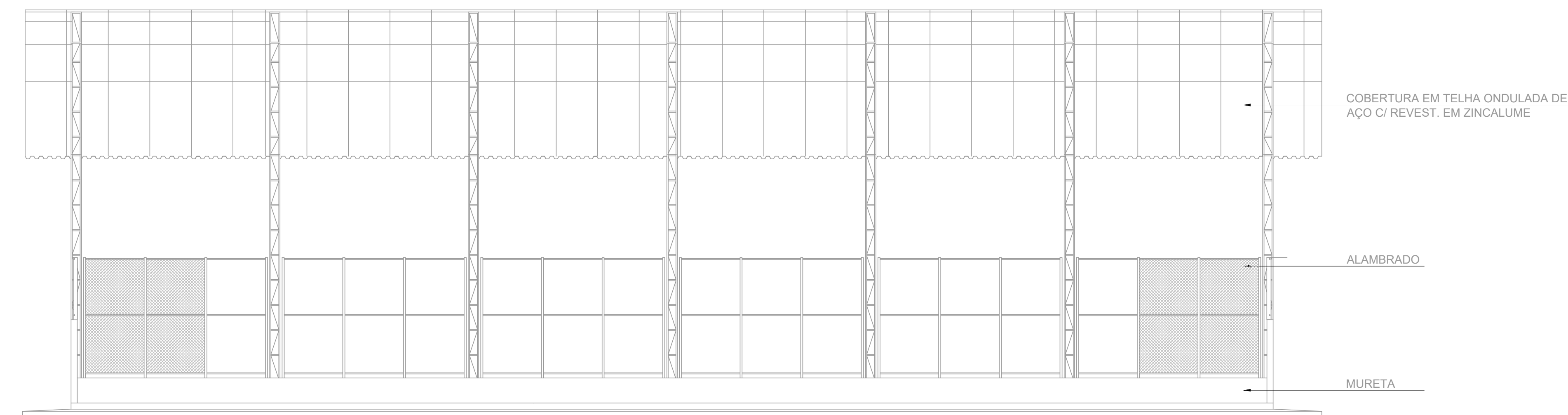
FACHADA LATERAL ESC.: 1/100
