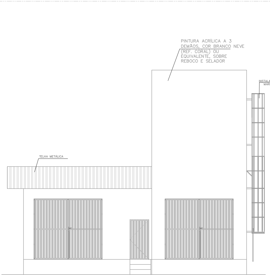
FACHADA ESC.: 1/100
