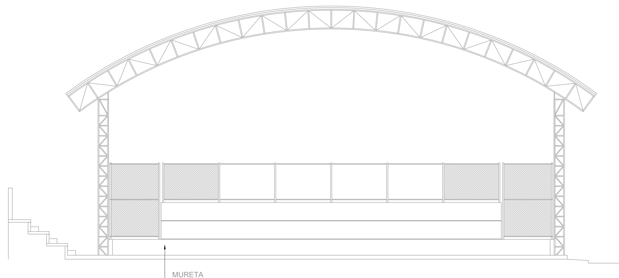
CORTE CD ESC.: 1/100
