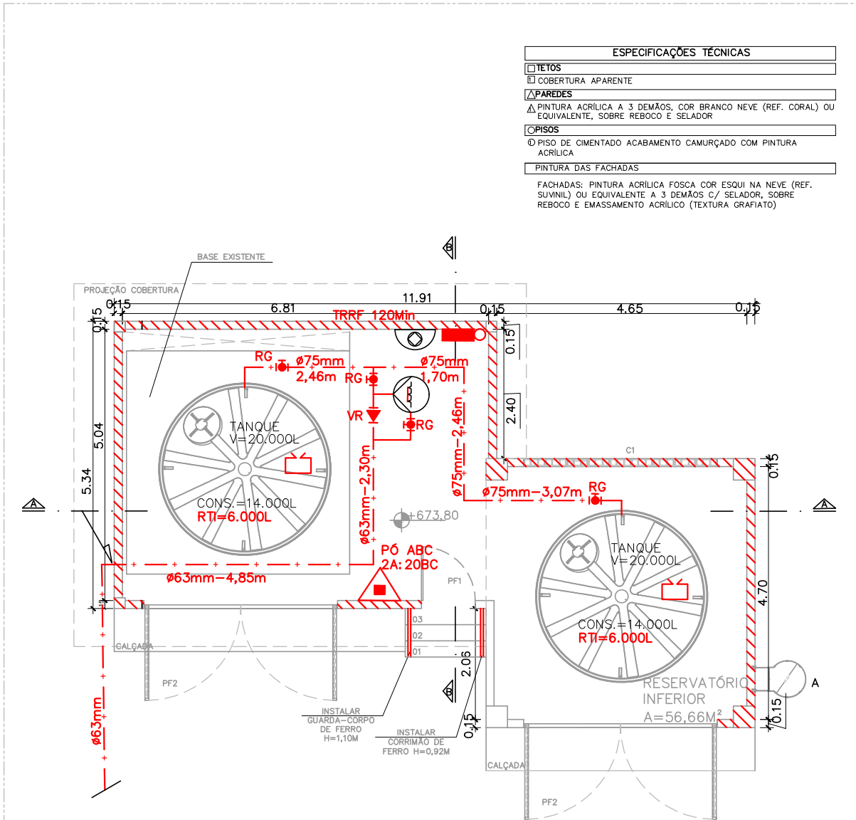
PLANTA BAIXA RESERVATÓRIOS INFERIORES ESC.: 1/100
