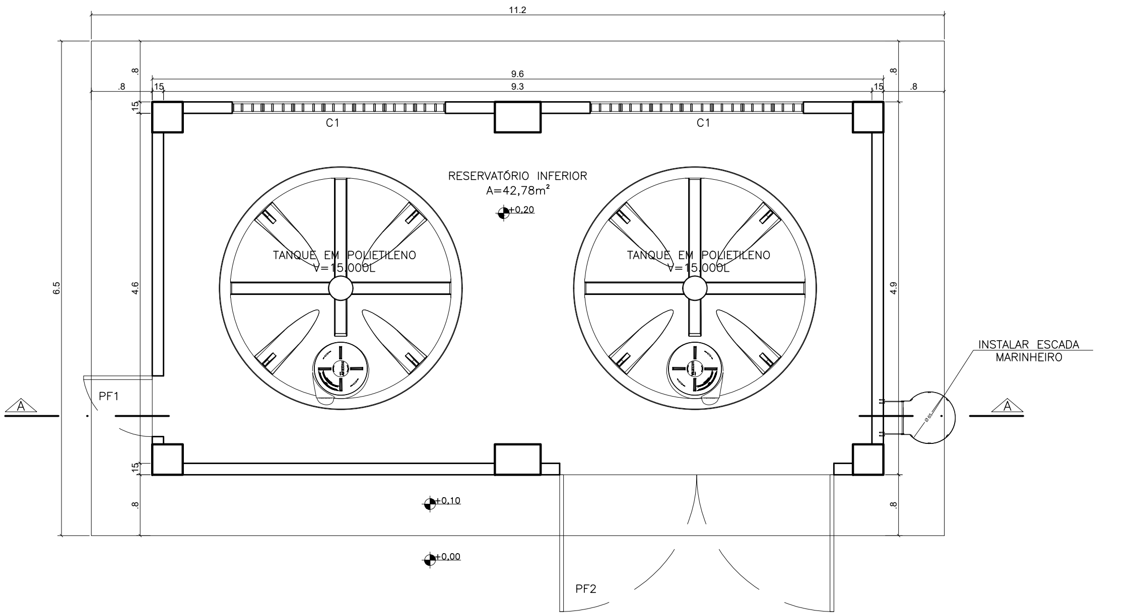
PLANTA BAIXA – RESERVATÓRIO INFERIOR ESC 1/50
