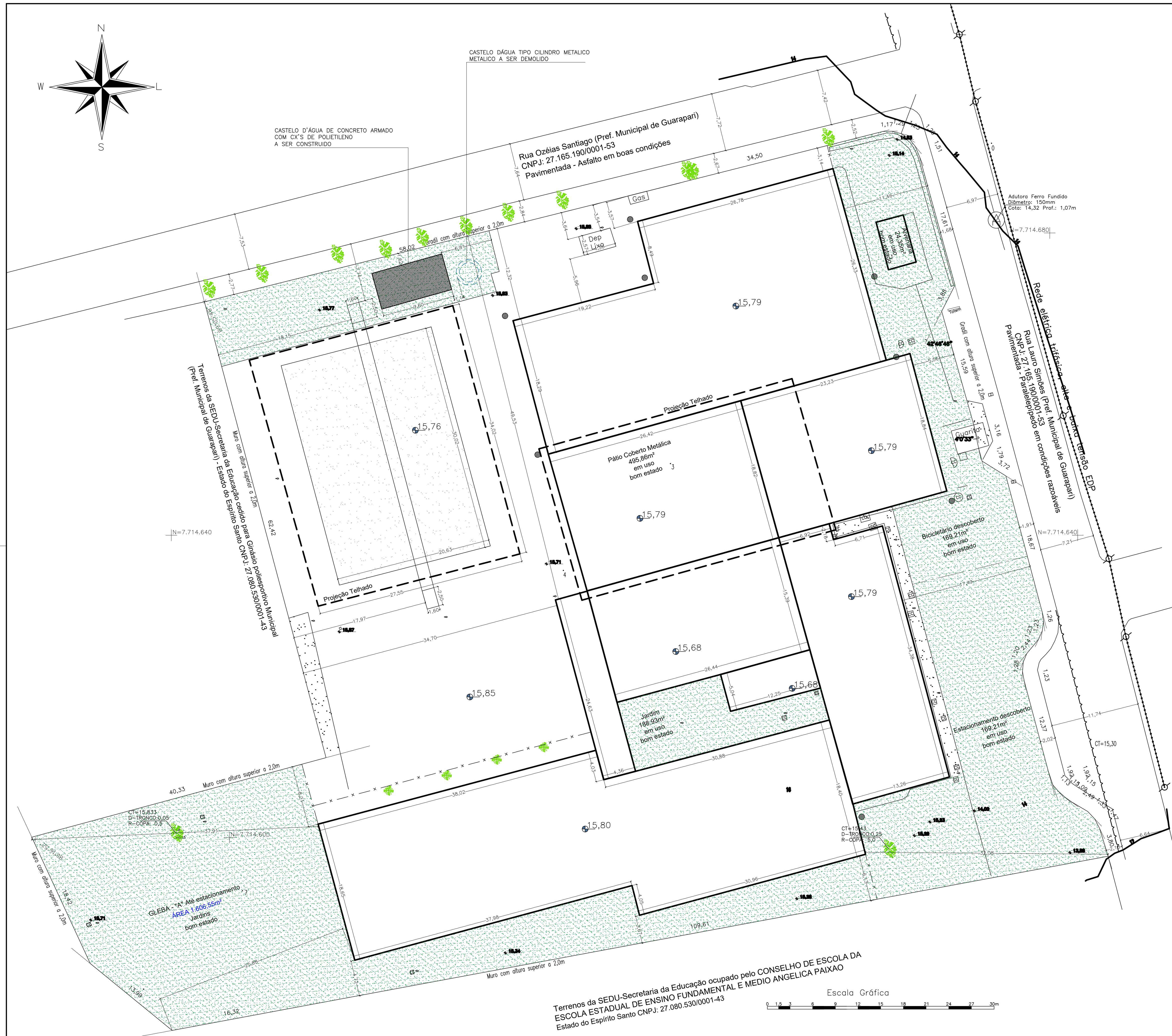
PLANTA DE IMPLANTAÇÃO – PROPOSTA ESC.:1/200
