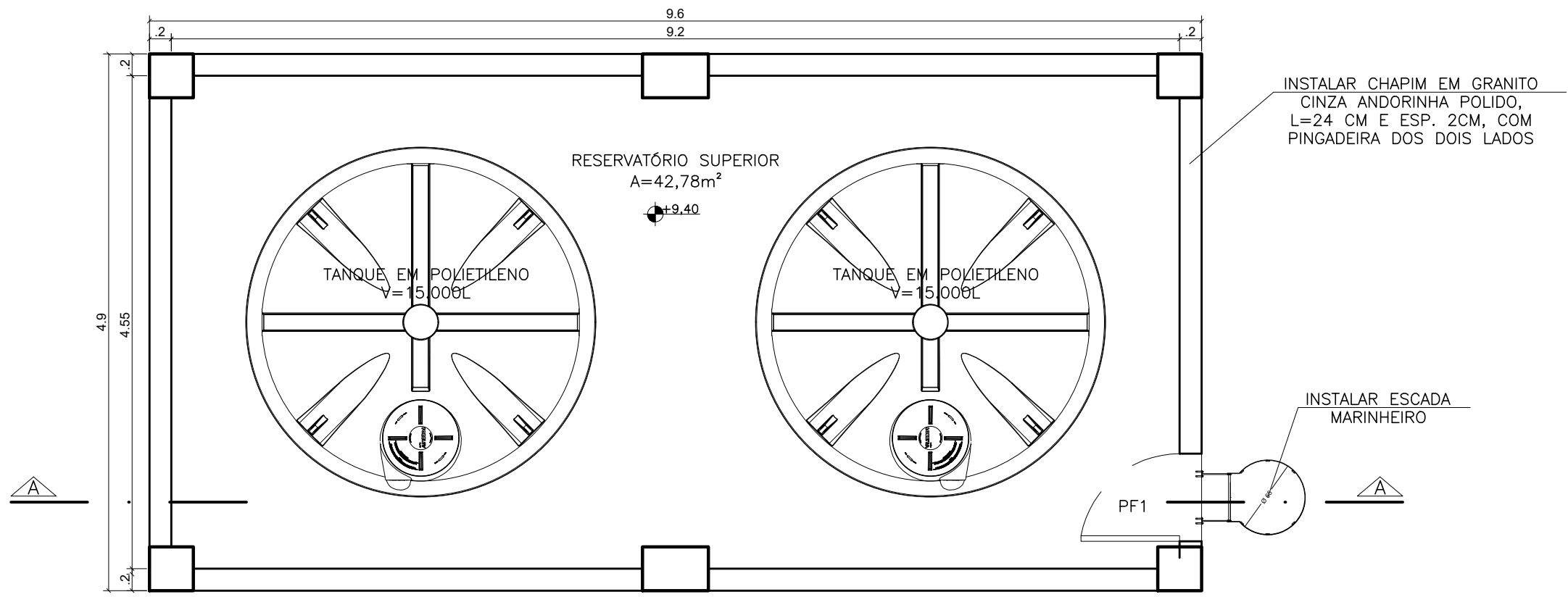
PLANTA BAIXA – RESERVATÓRIO SUPERIOR ESC 1/50
