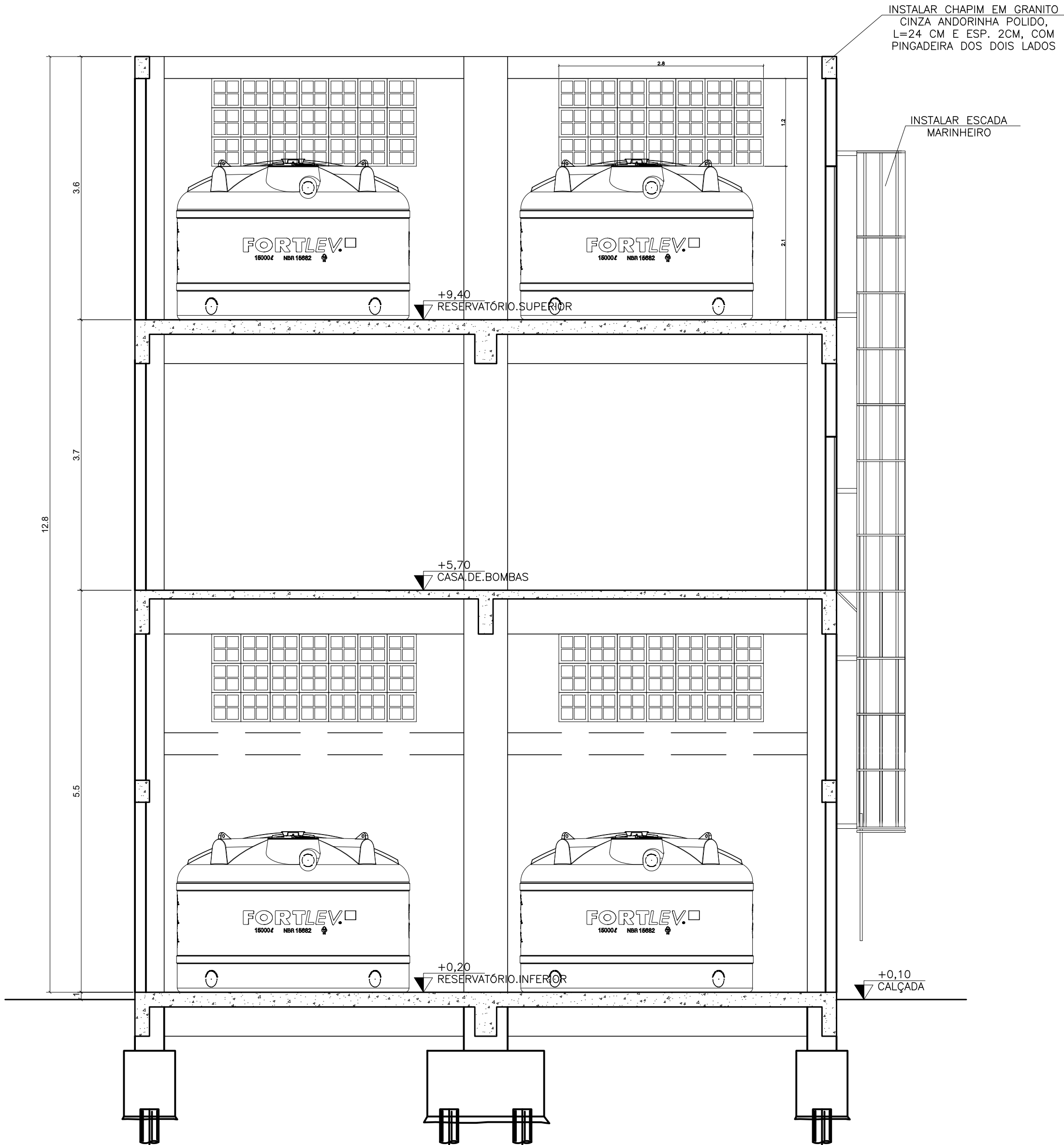
CORTE AA ESC 1/50
