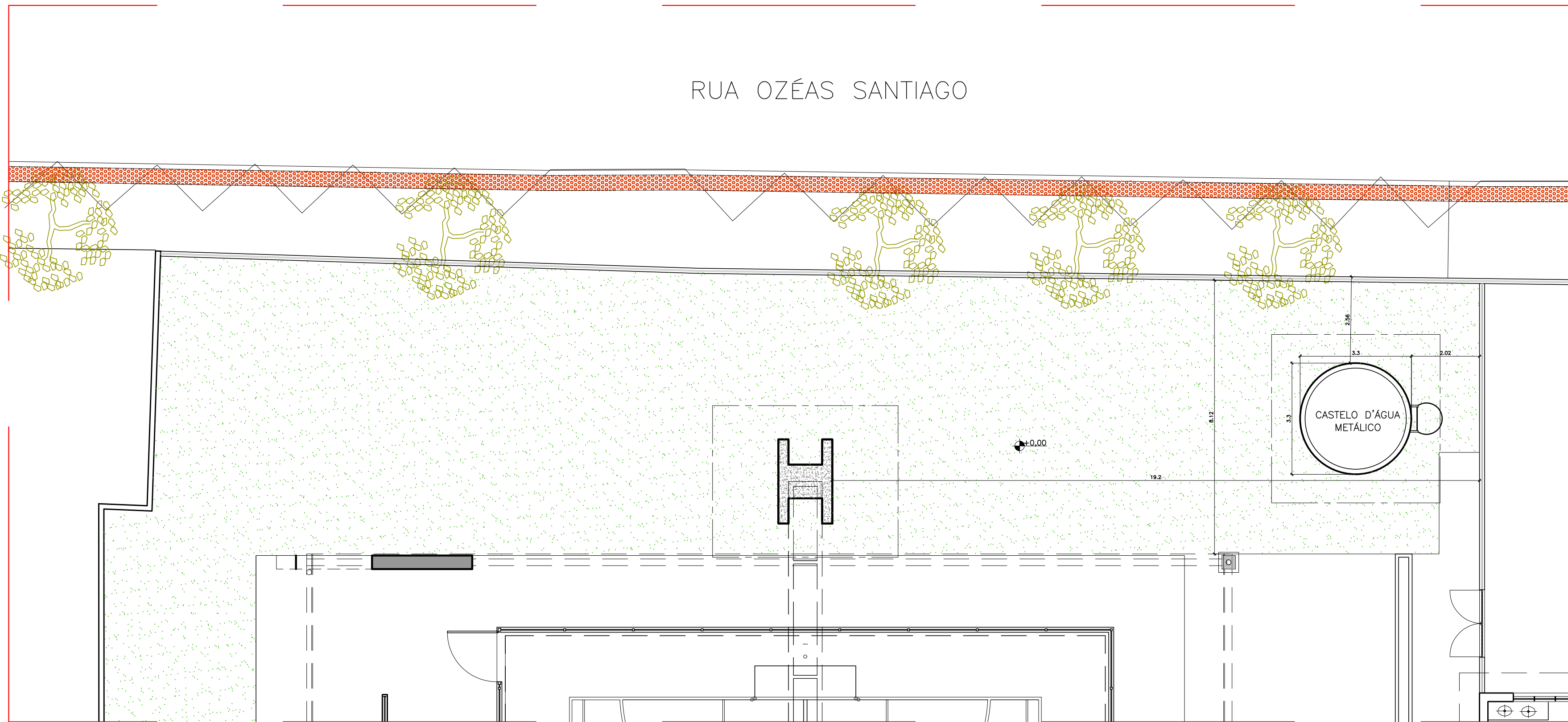
PLANTA DE IMPLANTAÇÃO - EXISTENTE ESC.:1/100
