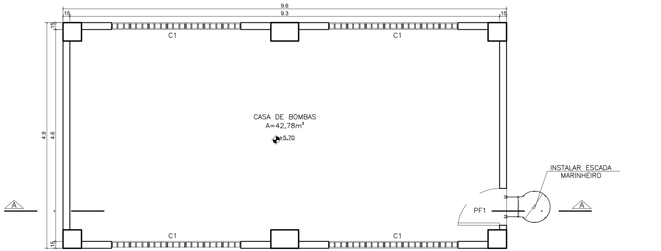
PLANTA BAIXA – CASA BOMBAS ESC 1/50
