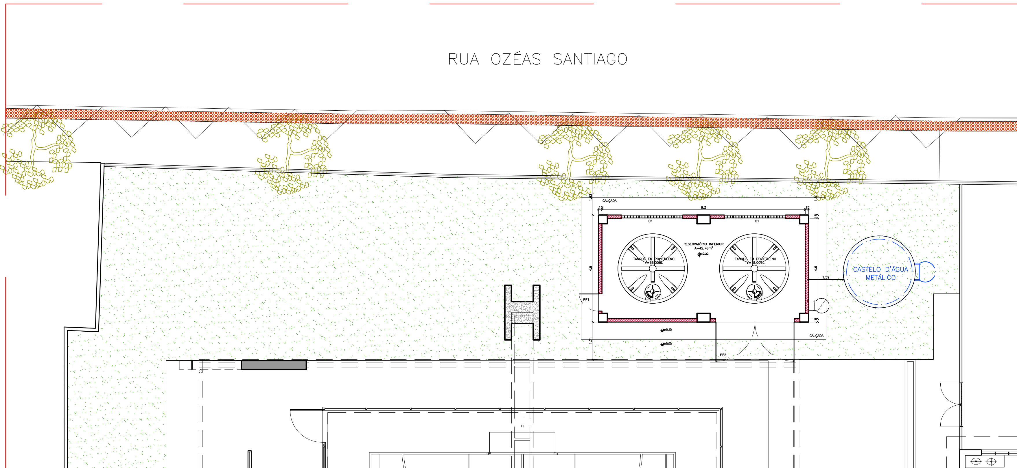
PLANTA DE IMPLANTAÇÃO - DEMOLIR/CONSTRUIR ESC.:1/100
