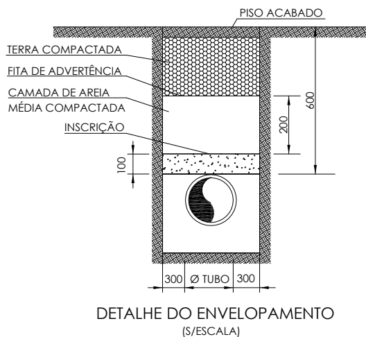
DETALHE 2 - ENVELOPE UTILIZANDO PLACA DE CONCRETO ARMADO (NOTA 2)
