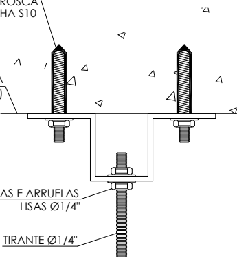
DETALHE 1 (S/ESCALA)
