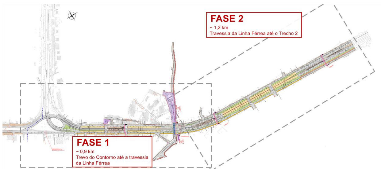
Figura 1 – Trecho 1 do CMN, com a divisão em Fase 1 e Fase 2. Fonte: Anteprojeto Geométrico (SEMOBI).
