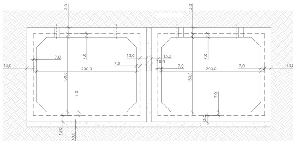
Figura 2: Seção BDCC 1,50 x 1,50 m proposto
