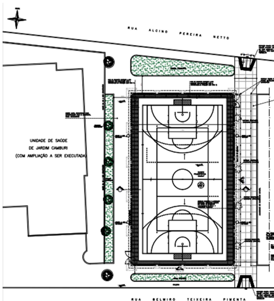
Figura 2 – Planta Baixa do projeto arquitetônico (Fonte: Projeto Arquitetônico)
