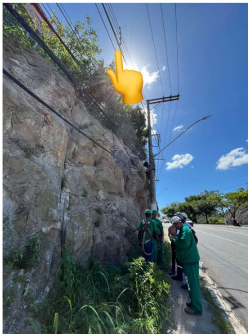
Figura 03 – Identificação da rede a ser isolada.
