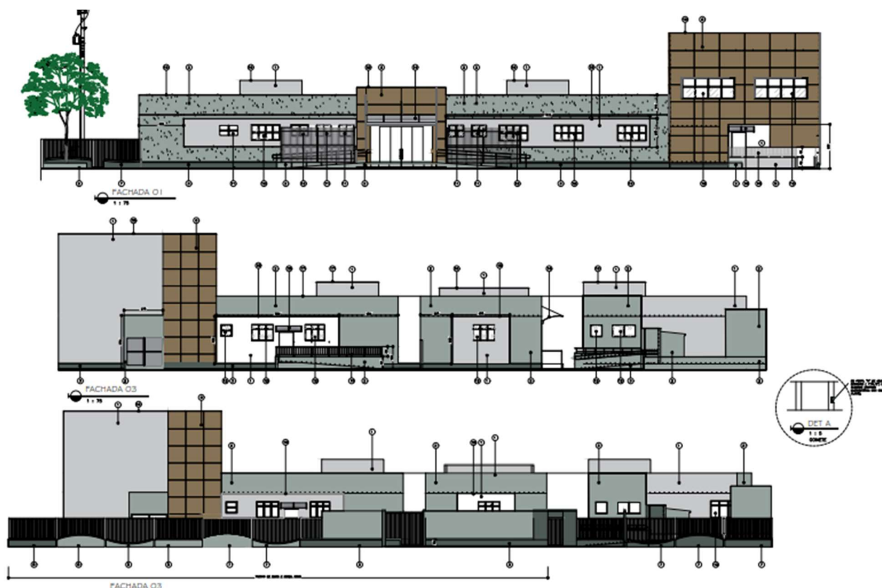
Figura 3 – Imagens das Fachadas do Projeto Arquitetônico da US Jardim Camburi
